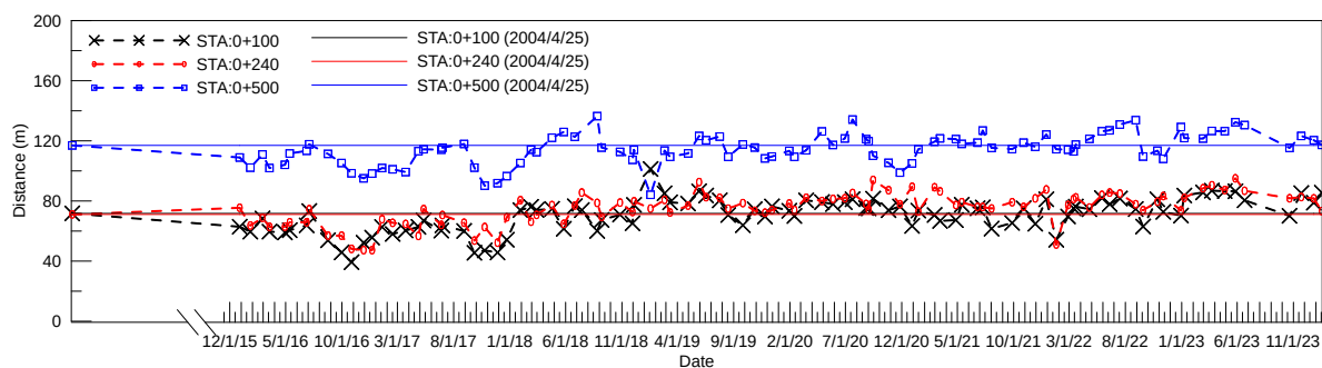
圖 4-21 岸線斷面沙灘寬度變化圖(2024/1/17)
