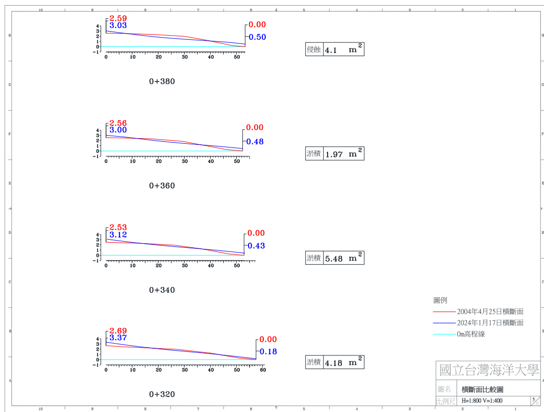
圖 4-4(f) 2024 年 1 月 17 日 A 監測區橫斷面比較圖
