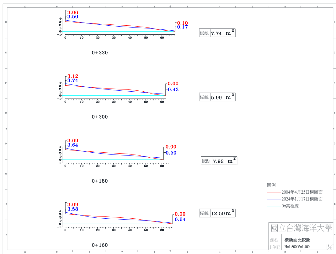
圖 4-4(h) 2024 年 1 月 17 日 A 監測區橫斷面比較圖
