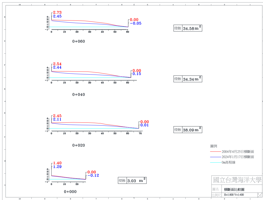
圖 4-4(j) 2024 年 1 月 17 日 A 監測區橫斷面比較圖
