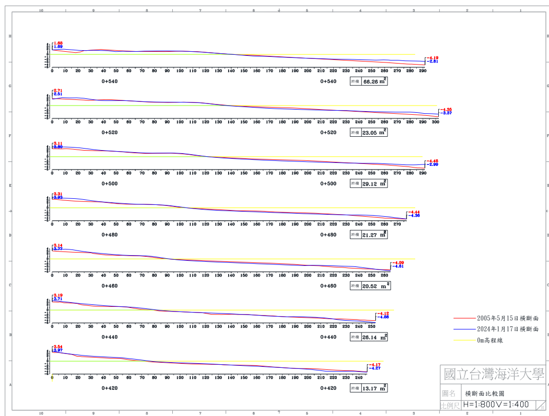
圖 4-5(c) 2024 年 1 月 17 日 B 監測區橫断面比較圖
