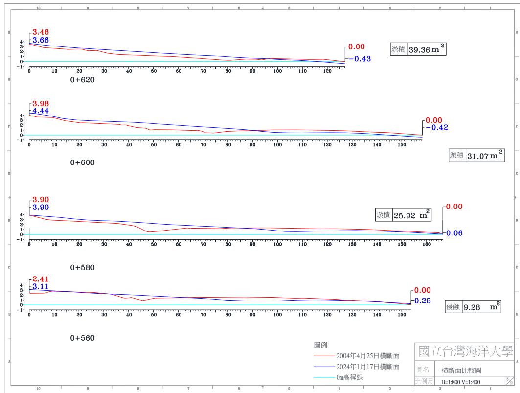
圖 4-4(c) 2024 年 1 月 17 日 A 監測區橫斷面比較圖
