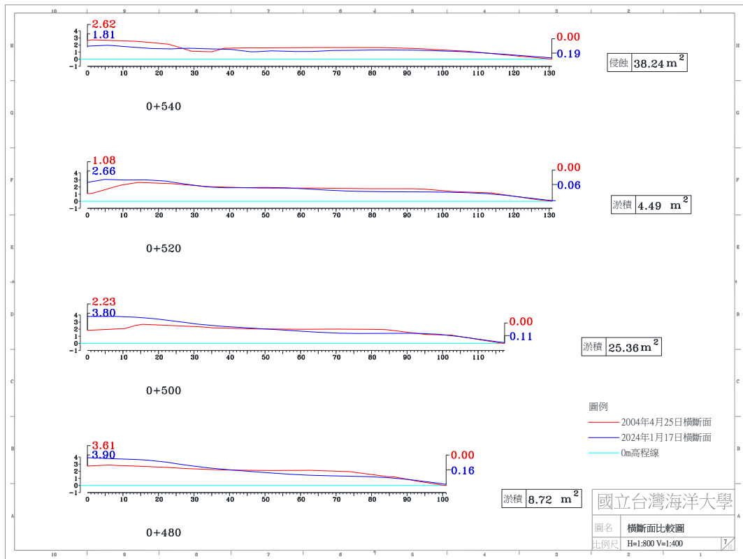
圖 4-4(d) 2024 年 1 月 17 日 A 監測區橫斷面比較圖
