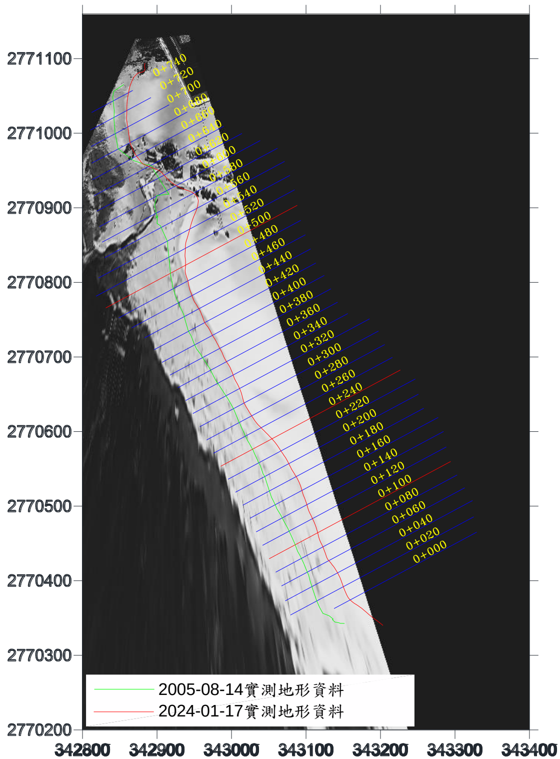
圖 4-22 長期實測 0 m 灘線比對平面示意圖
