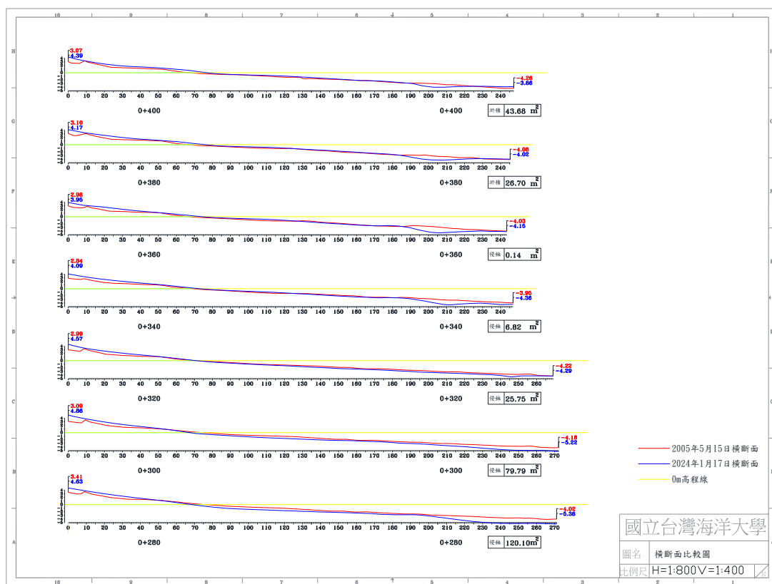
圖 4-5(d) 2024 年 1 月 17 日 B 監測區橫断面比較圖
