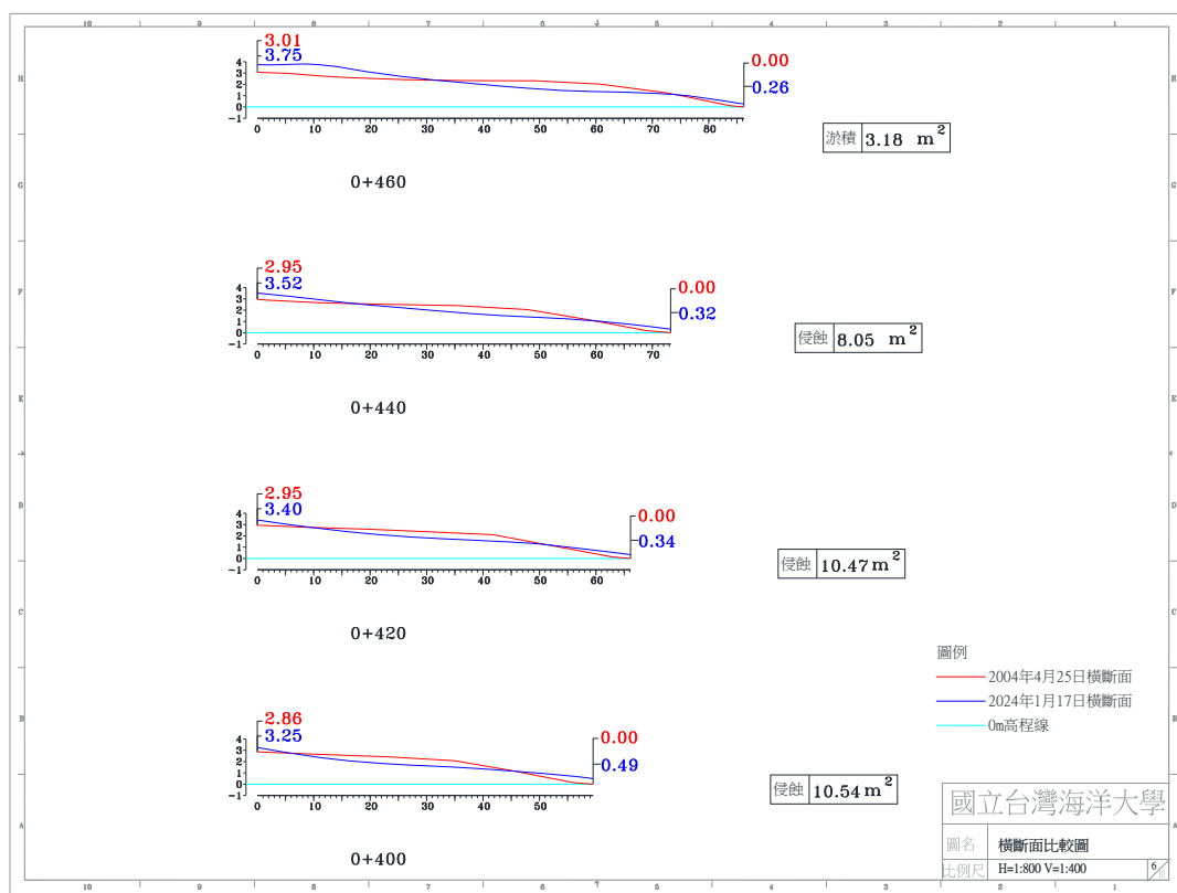
圖 4-4(e) 2024 年 1 月 17 日 A 監測區橫斷面比較圖
