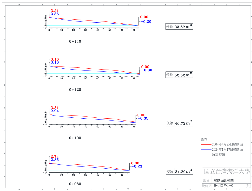
圖 4-4(i) 2024 年 1 月 17 日 A 監測區橫斷面比較圖
