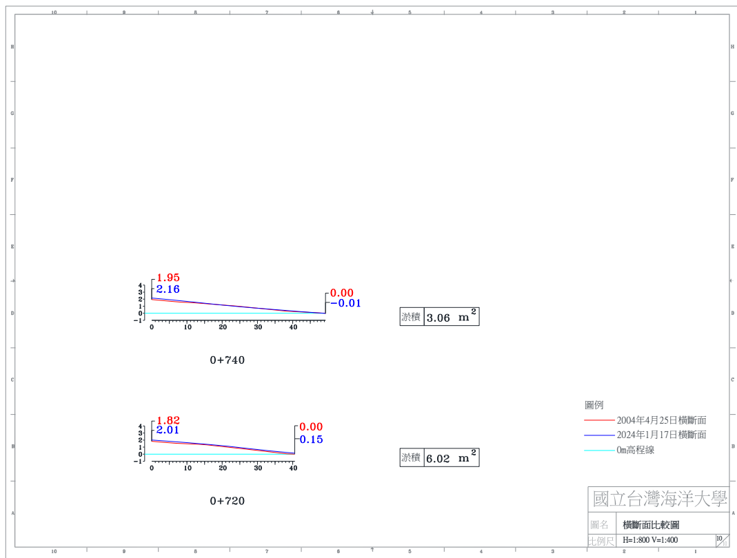
圖 4-4(a) 2024 年 1 月 17 日 A 監測區橫斷面比較圖
