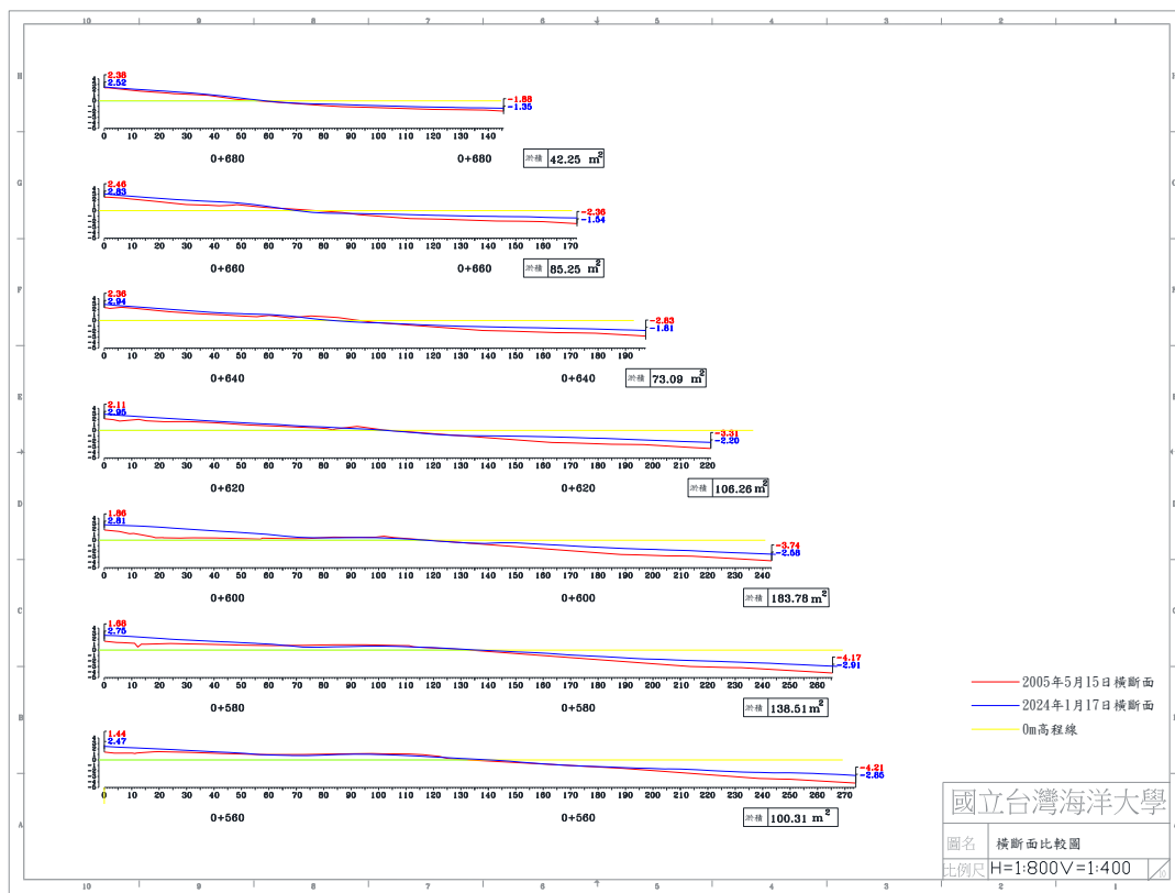
圖 4-5(b) 2024 年 1 月 17 日 B 監測區橫斷面比較圖
