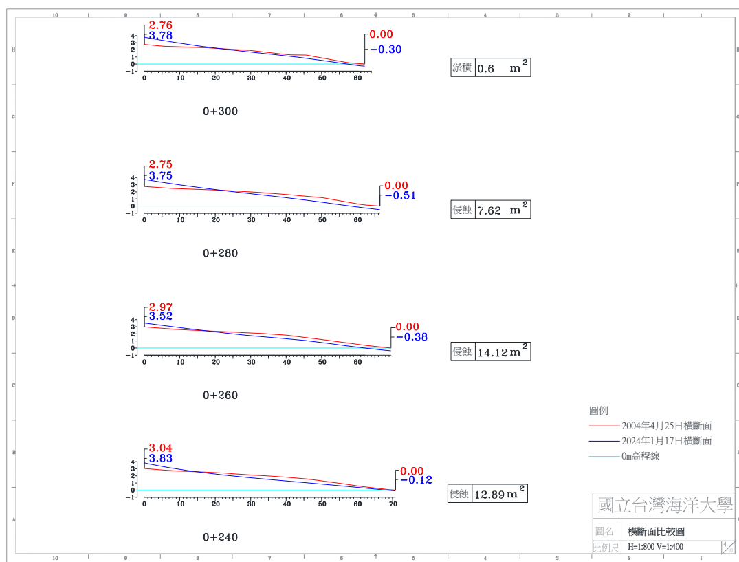
圖 4-4(g) 2024 年 1 月 17 日 A 監測區橫斷面比較圖
