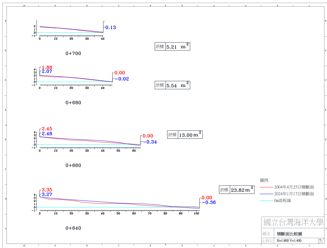
圖 4-4(b) 2024 年 1 月 17 日 A 監測區橫斷面比較圖
