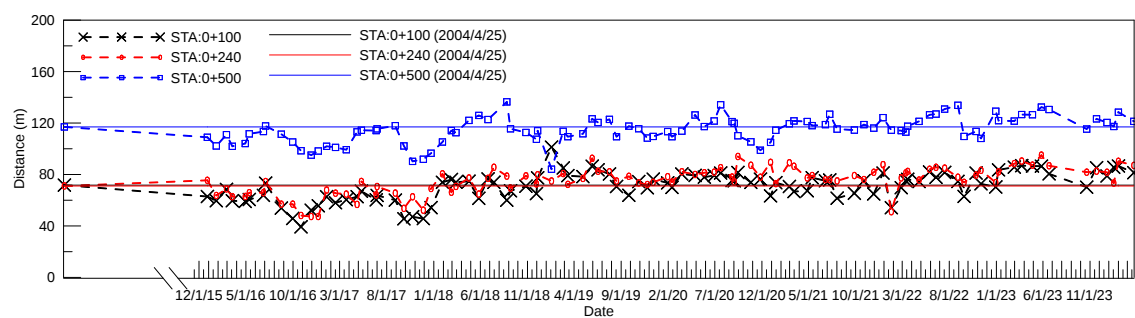
圖 4-16 海岸線斷面沙灘寬度變化圖(斷面編號：0+100、0+240、0+500)
