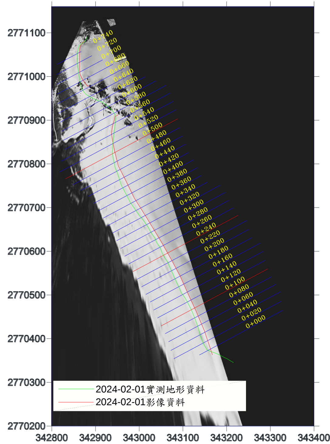
圖 3-21 水位線分析結果圖(2024/02/01)
