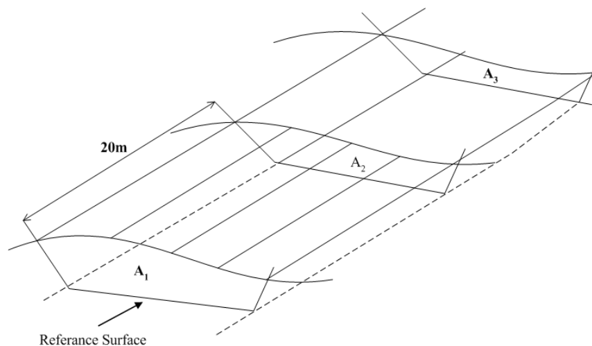
圖 3-4 土方計算原理示意圖
