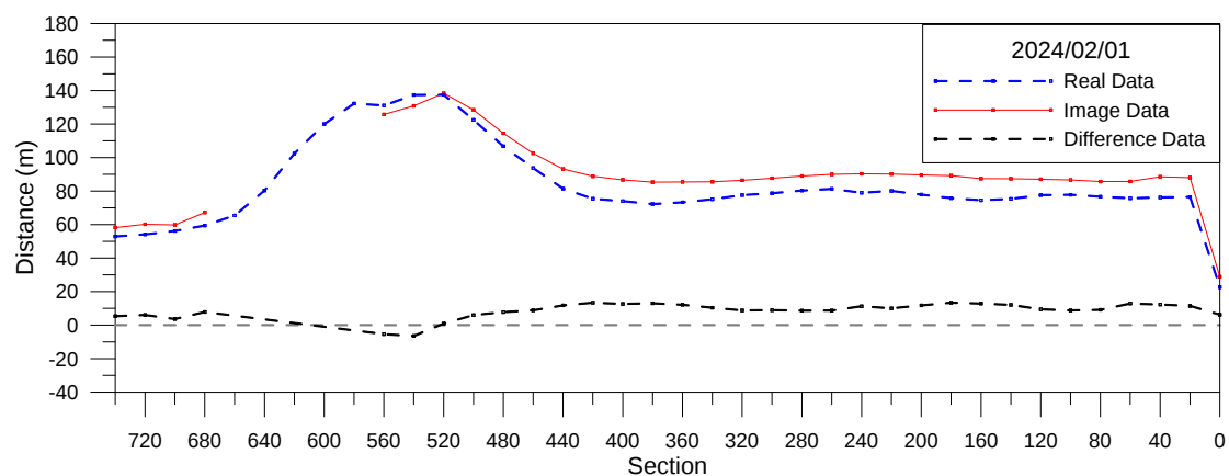
圖 3-22 海岸線分析比較圖(2024/02/01)
