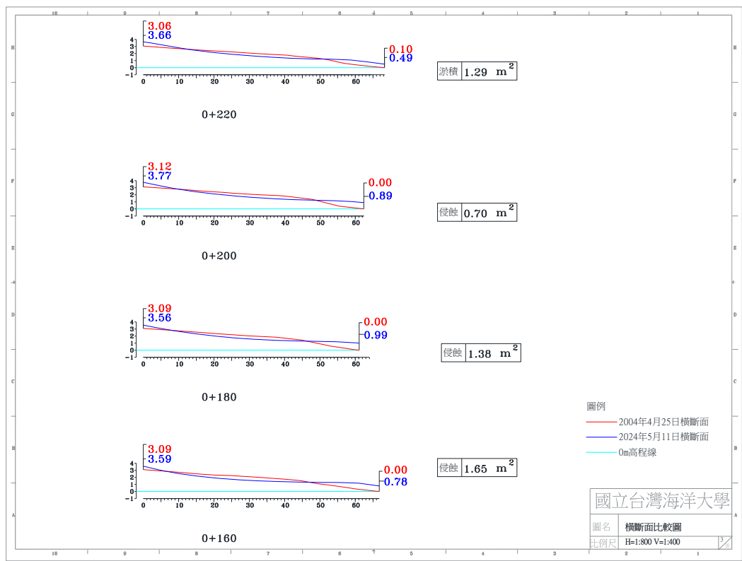
圖 4-4(h) 2024 年 5 月 11 日 A 監測區橫斷面比較圖
