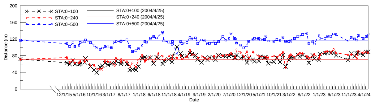
圖 4-21 岸線斷面沙灘寬度變化圖(2024/5/11)
