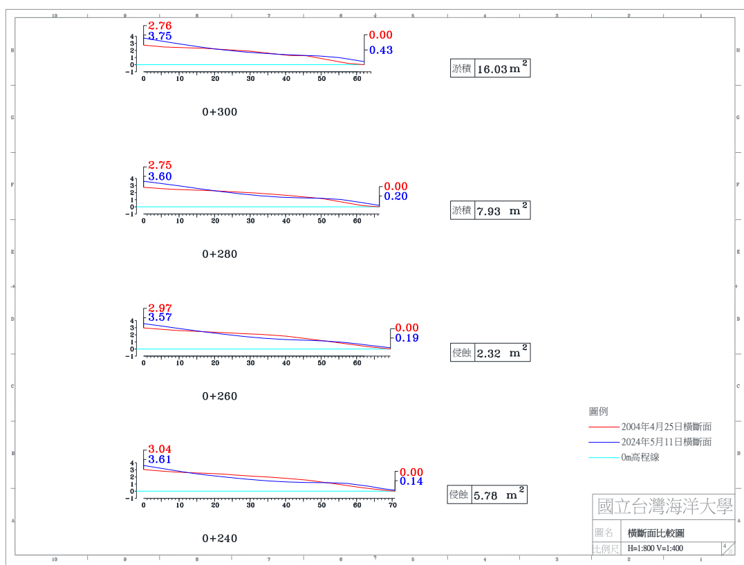
圖 4-4(g) 2024 年 5 月 11 日 A 監測區橫斷面比較圖
