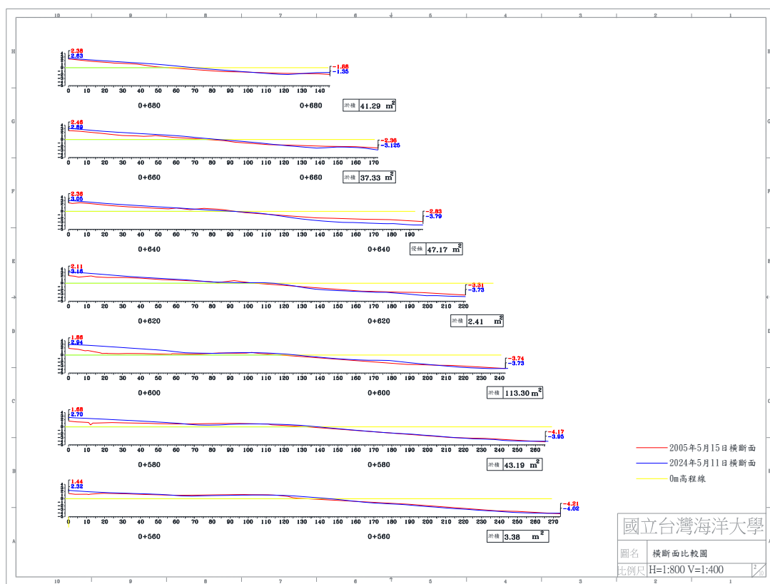
圖 4-5(b) 2024 年 5 月 11 日 B 監測區橫断面比較圖
