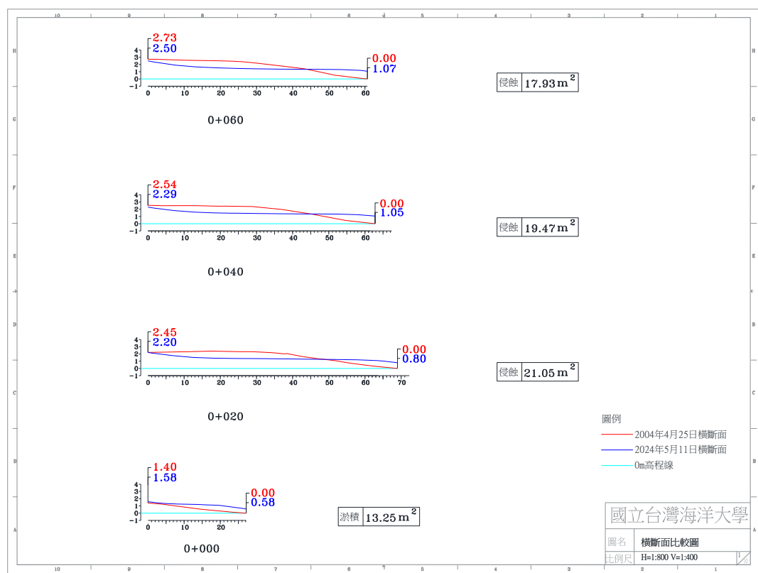
圖 4-4(j) 2024 年 5 月 11 日 A 監測區橫斷面比較圖
