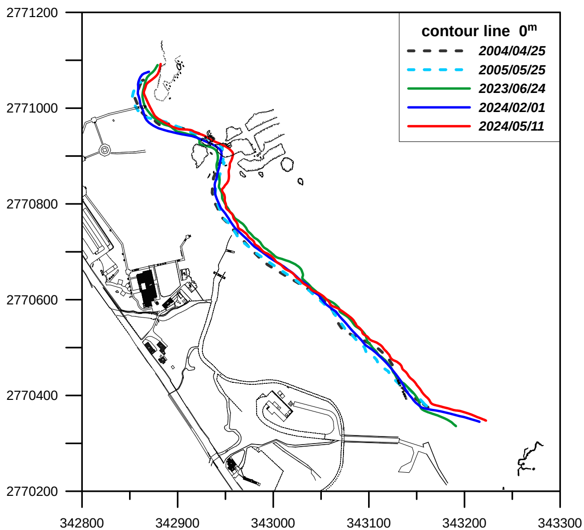
圖 4-2 監測區 0 m 岸線變化比較圖
