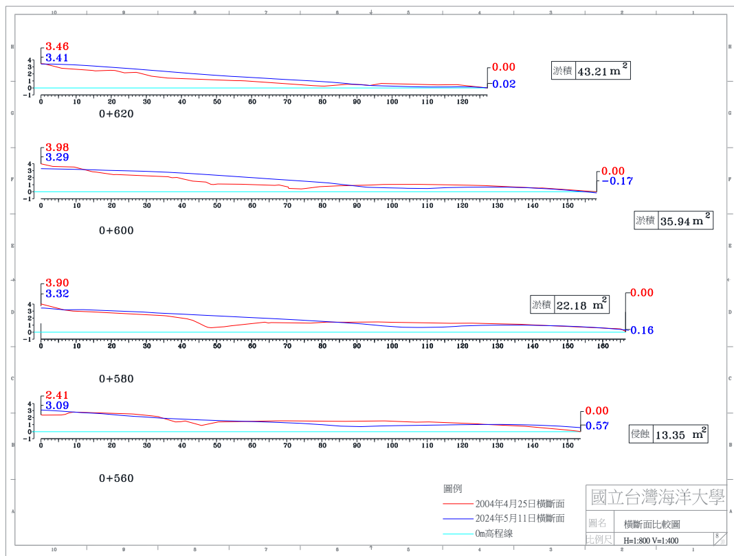
圖 4-4(c) 2024 年 5 月 11 日 A 監測區橫斷面比較圖
