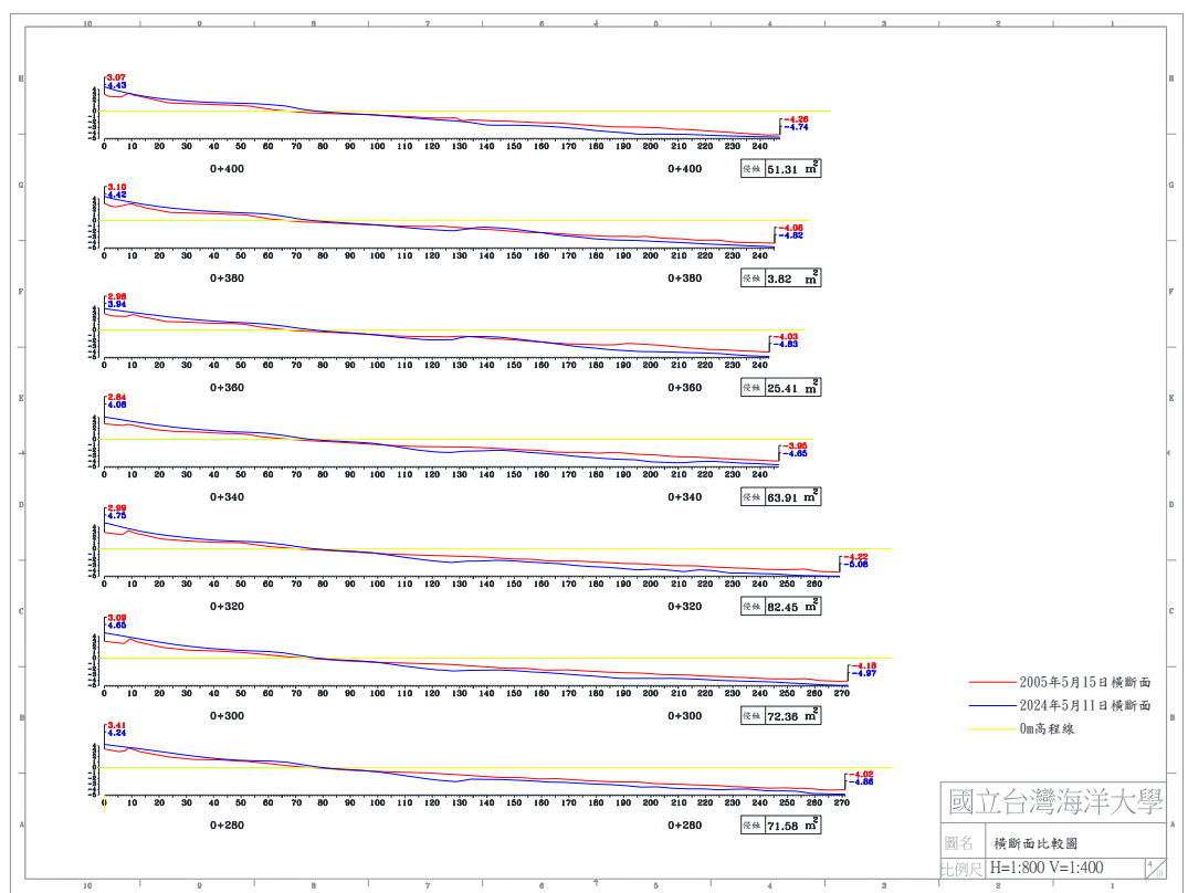
圖 4-5(d) 2024 年 5 月 11 日 B 監測區橫斷面比較圖
