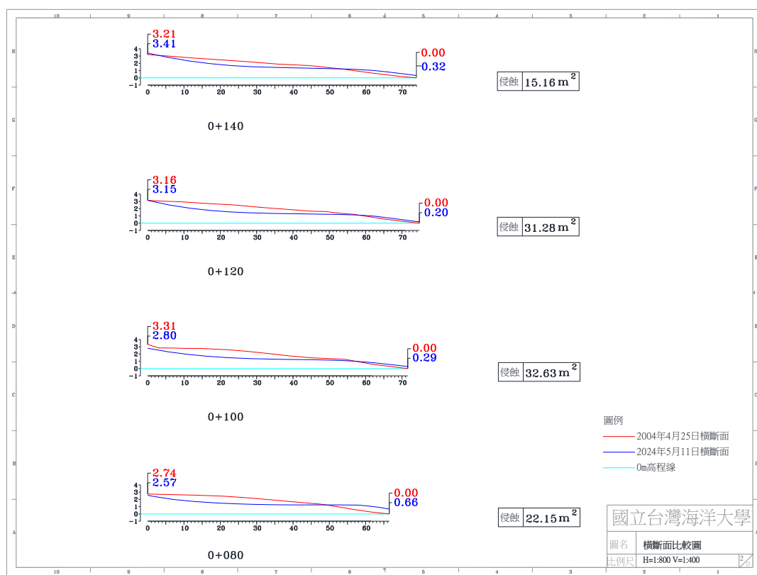
圖 4-4(i) 2024 年 5 月 11 日 A 監測區橫斷面比較圖
