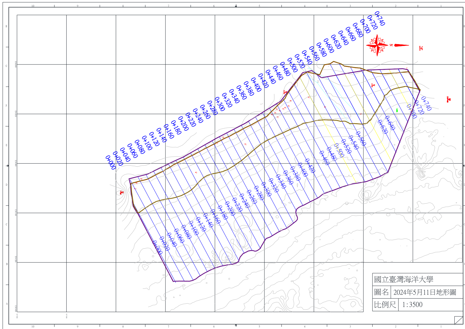
圖 4-1 2024 年 5 月 11 日監測地形
