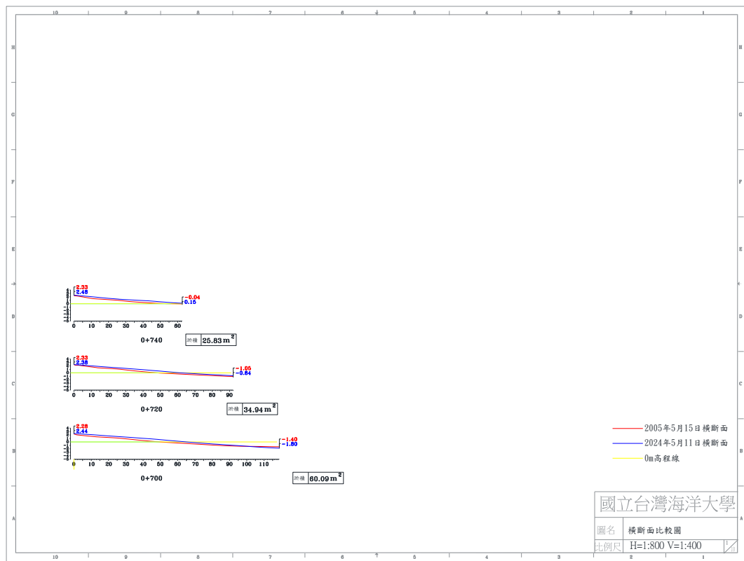
圖 4-5(a) 2024 年 5 月 11 日 B 監測區橫断面比較圖
