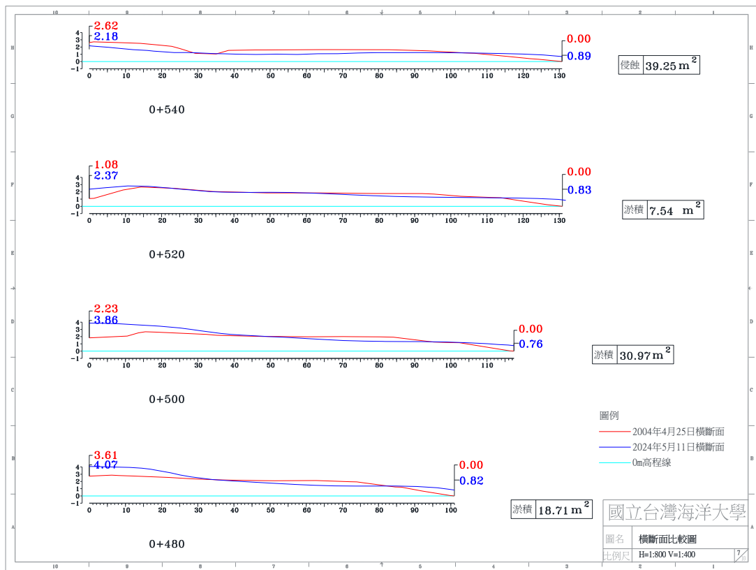
圖 4-4(d) 2024 年 5 月 11 日 A 監測區橫斷面比較圖
