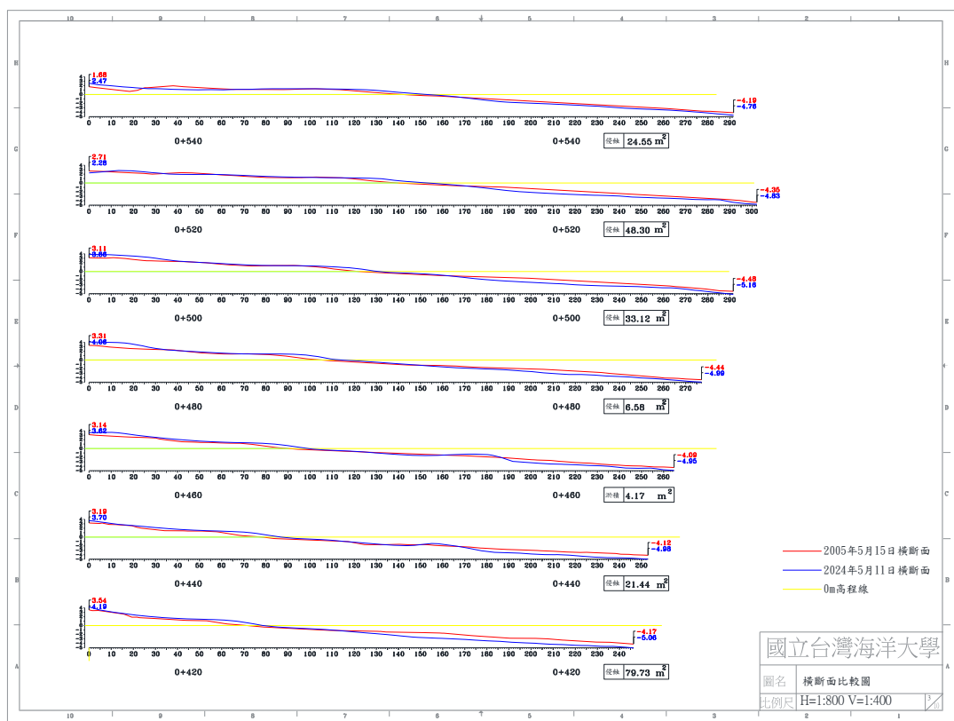
圖 4-5(c) 2024 年 5 月 11 日 B 監測區橫斷面比較圖
