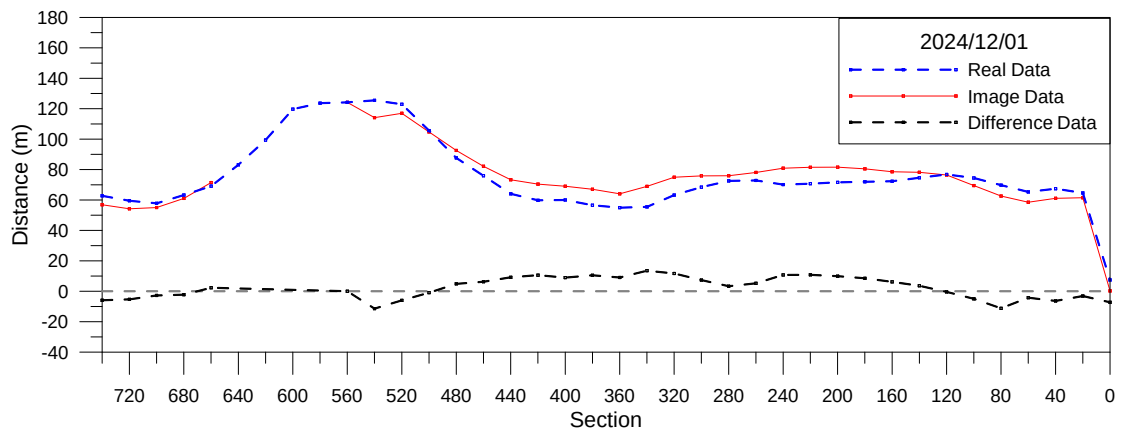
圖 3-22 海岸線分析比較圖(2024/12/01)
