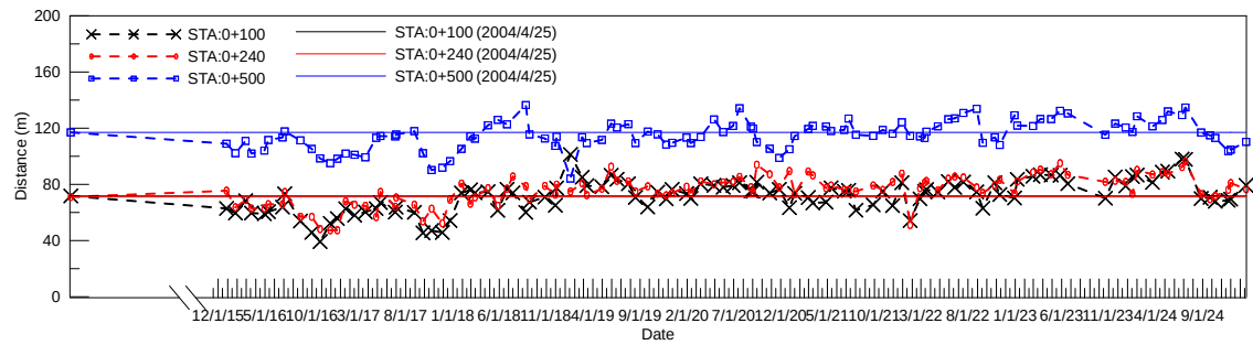
圖 4-16 岸線斷面沙灘寬度變化圖(2025/01/20)
