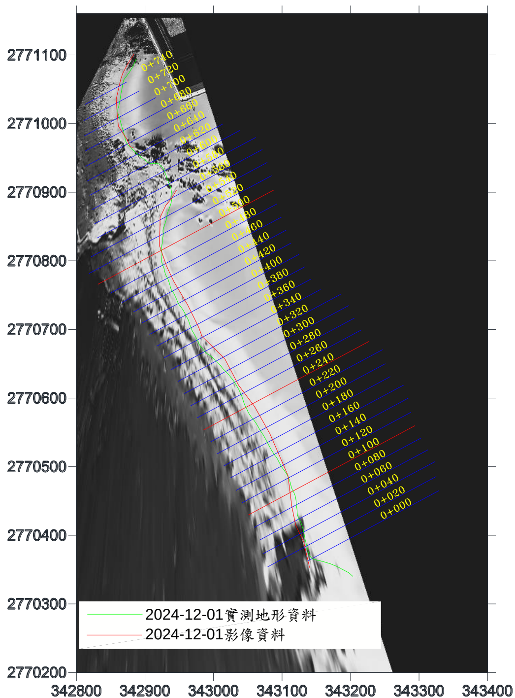
圖 3-21 水位線分析結果圖(2024/12/01)
