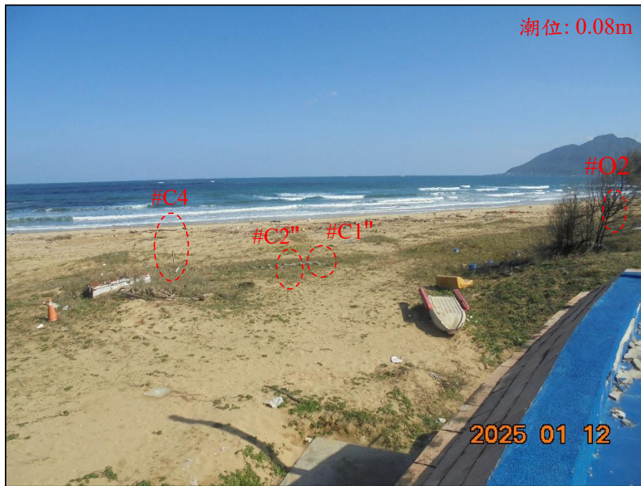
附圖 2-5 小舞台南側輔助觀測樁位置圖(2025/01/12)
