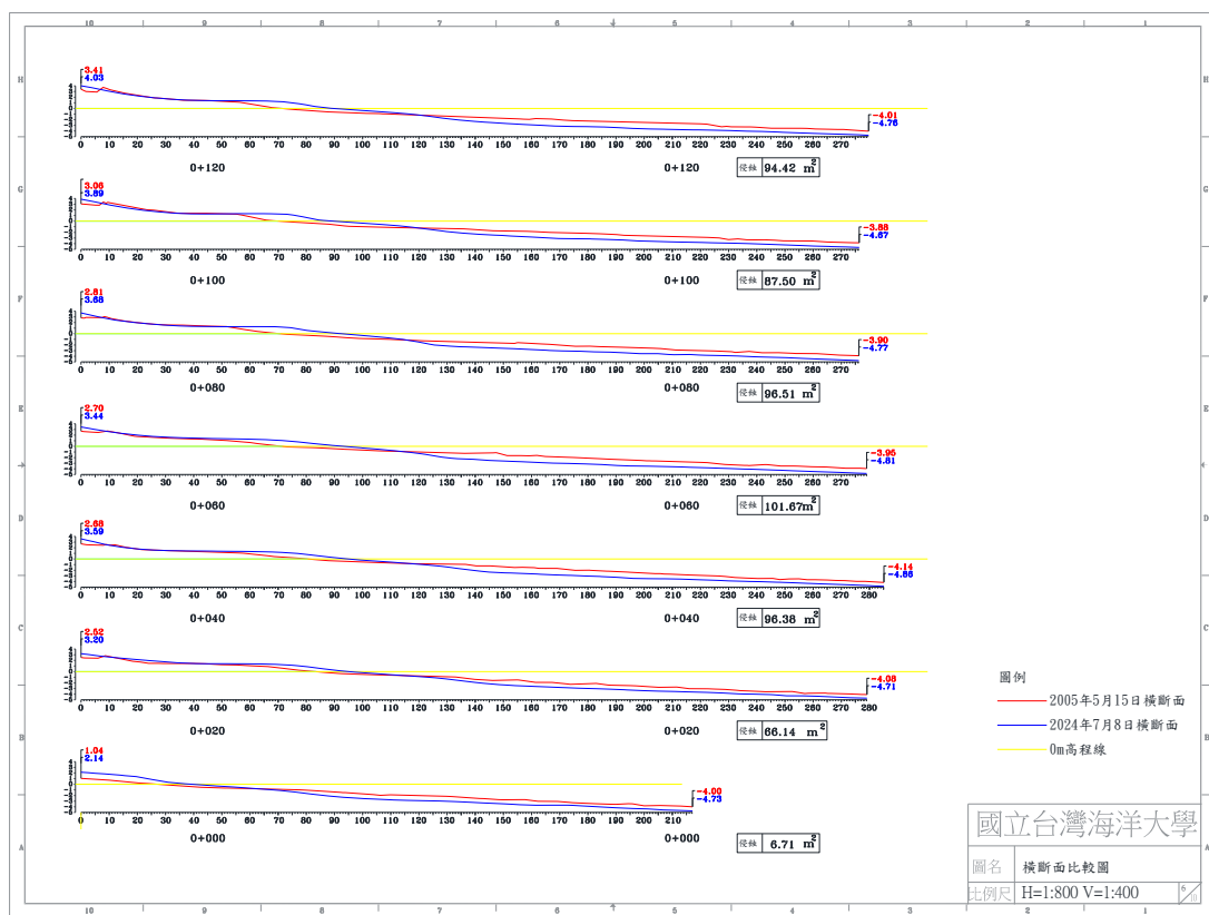
圖 4-5(f) 2024 年 7 月 8 日 B 監測區橫断面比較圖
