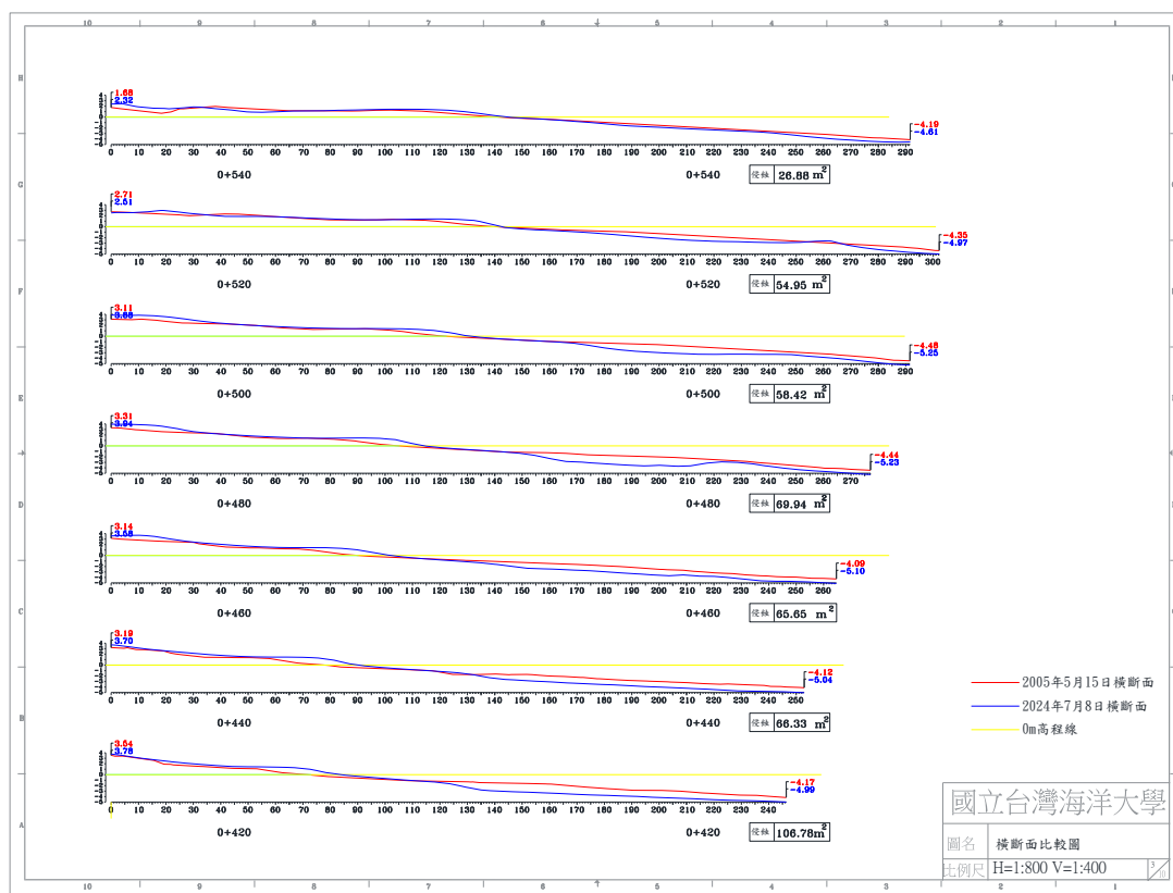
圖 4-5(c) 2024 年 7 月 8 日 B 監測區橫斷面比較圖
