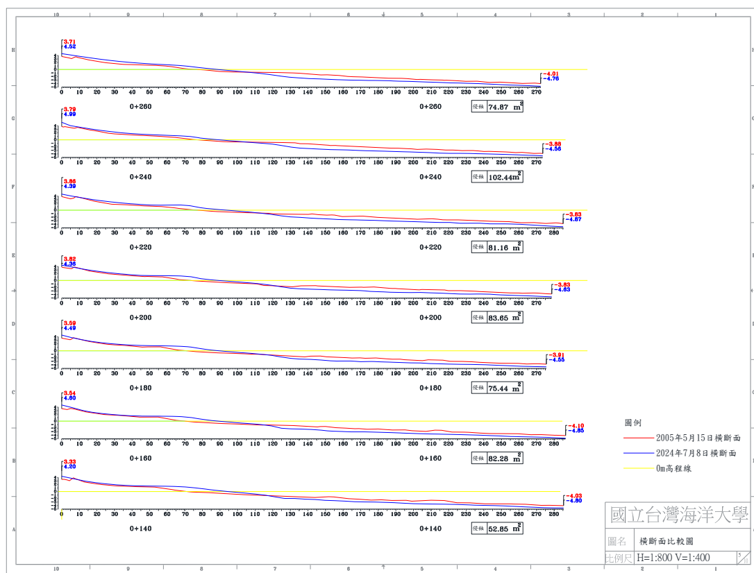
圖 4-5(e) 2024 年 7 月 8 日 B 監測區橫断面比較圖
