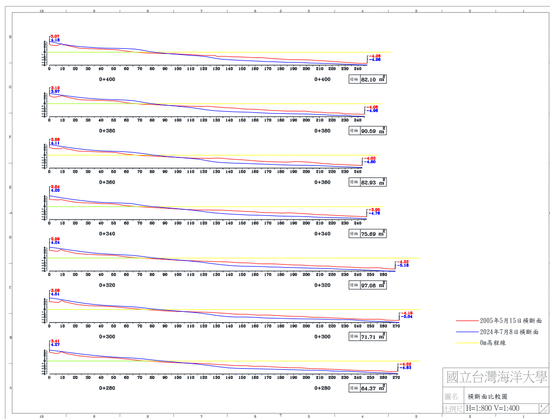
圖 4-5(d) 2024 年 7 月 8 日 B 監測區橫斷面比較圖
