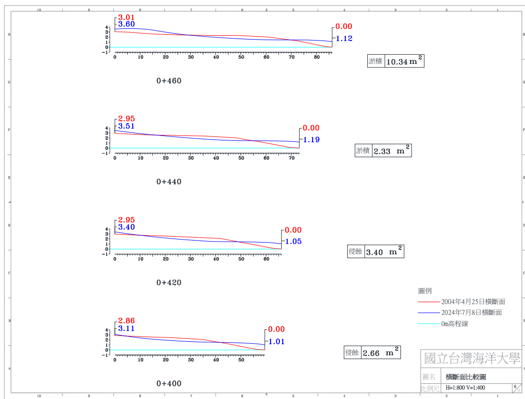
圖 4-4(e) 2024 年 7 月 8 日 A 監測區橫斷面比較圖
