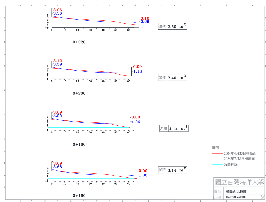
圖 4-4(h) 2024 年 7 月 8 日 A 監測區橫斷面比較圖
