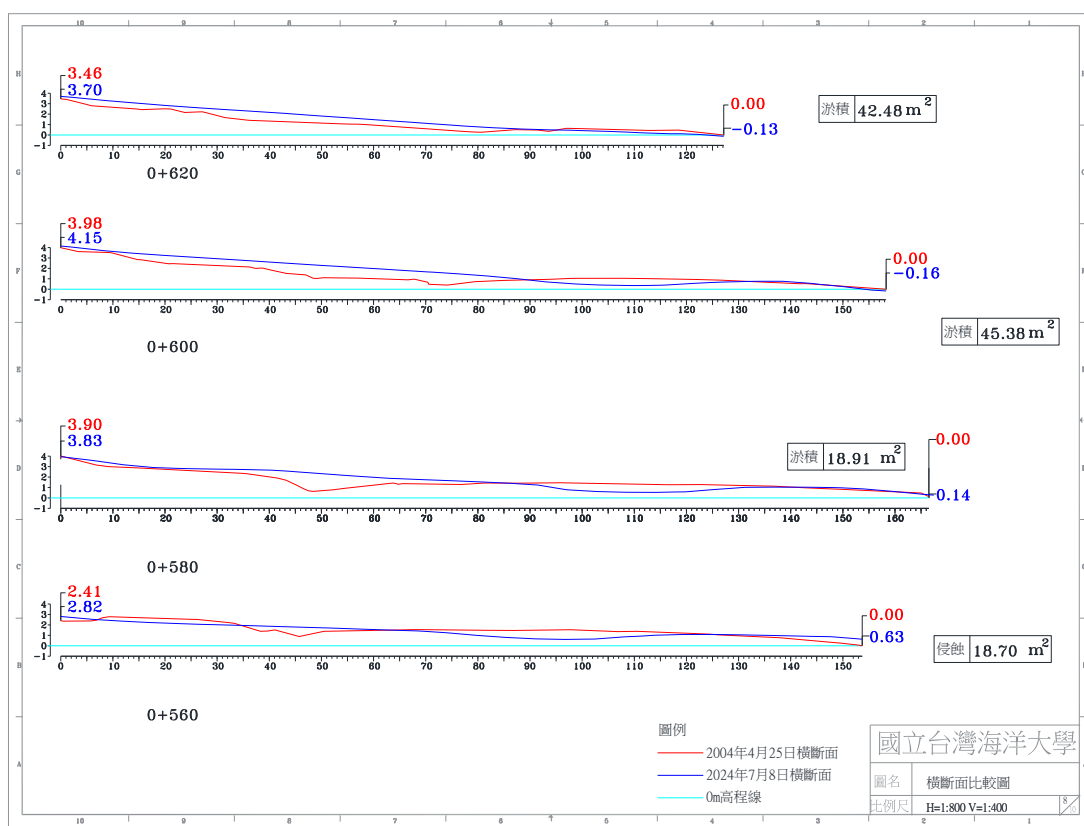
圖 4-4(c) 2024 年 7 月 8 日 A 監測區橫斷面比較圖
