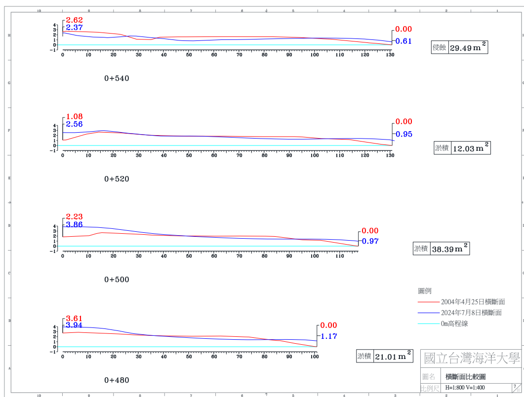
圖 4-4(d) 2024 年 7 月 8 日 A 監測區橫斷面比較圖
