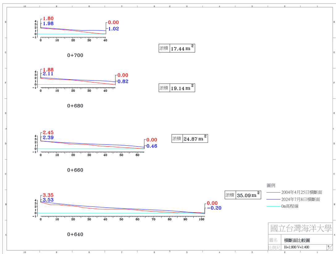
圖 4-4(b) 2024 年 7 月 8 日 A 監測區橫斷面比較圖
