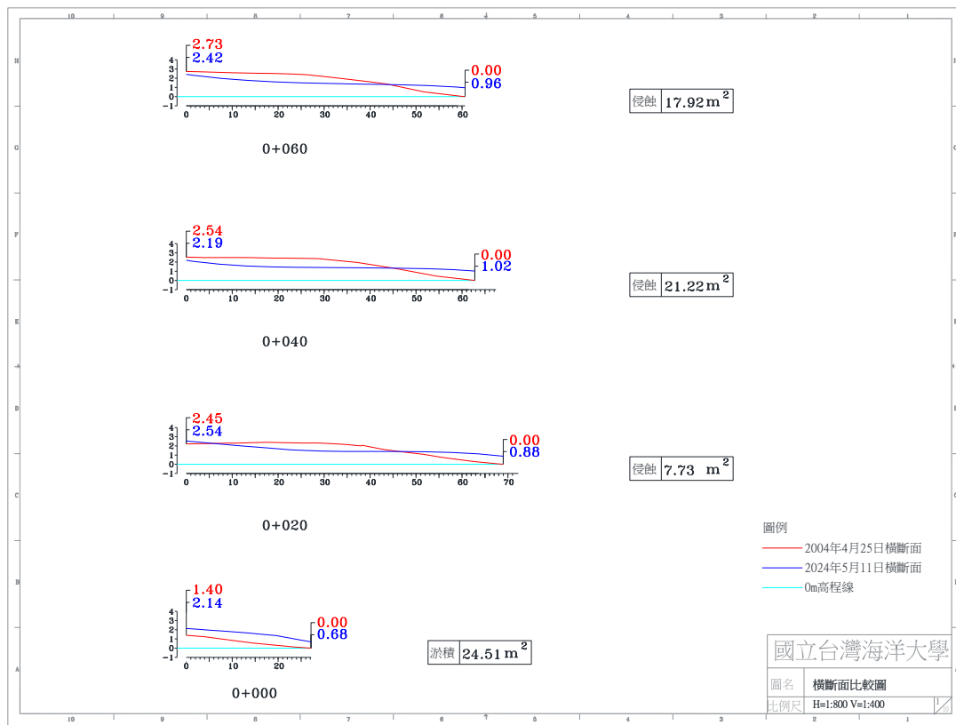
圖 4-4(j) 2024 年 7 月 8 日 A 監測區橫斷面比較圖
