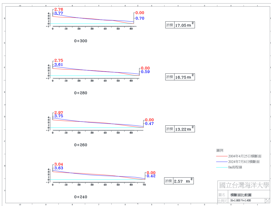
圖 4-4(g) 2024 年 7 月 8 日 A 監測區橫斷面比較圖
