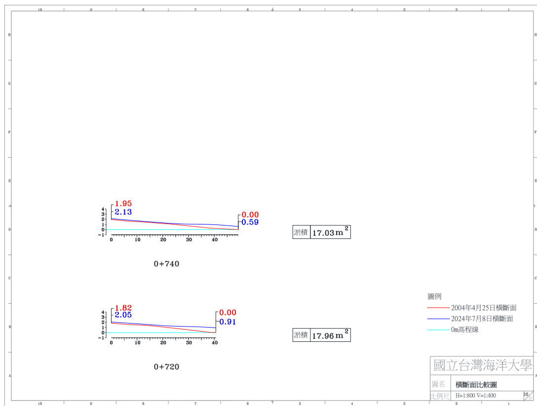
圖 4-4(a) 2024 年 7 月 8 日 A 監測區橫斷面比較圖
