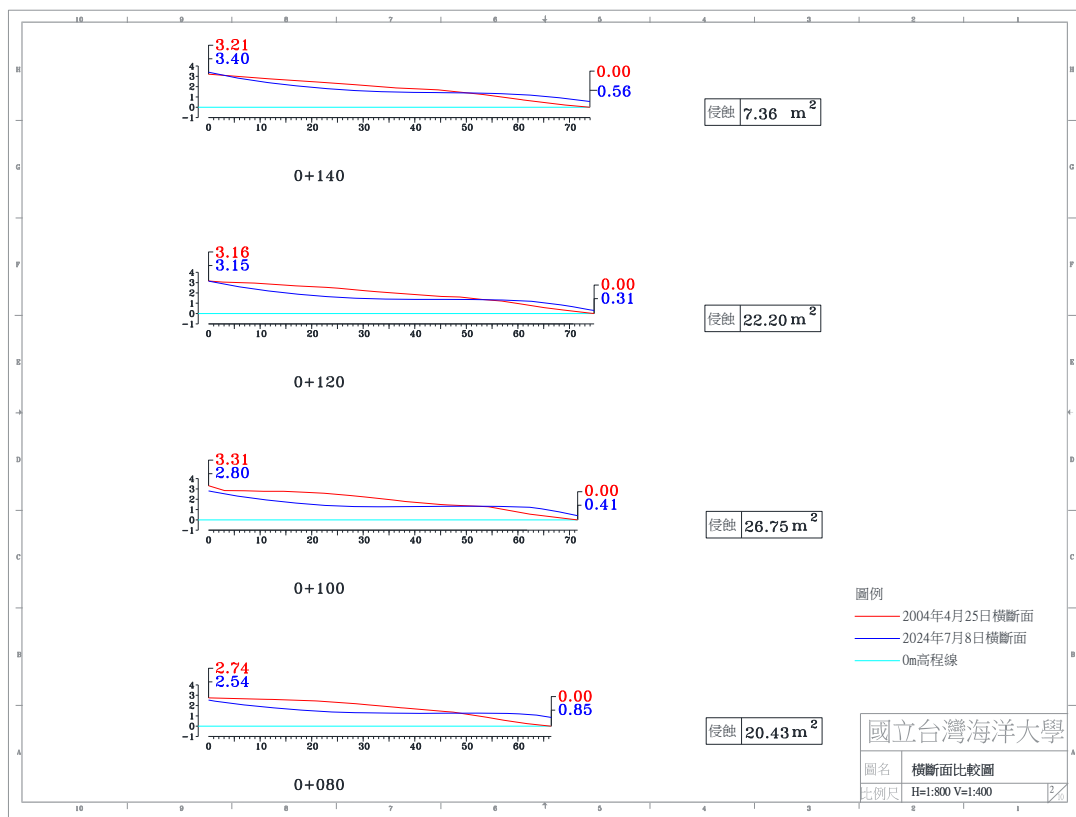
圖 4-4(i) 2024 年 7 月 8 日 A 監測區橫斷面比較圖
