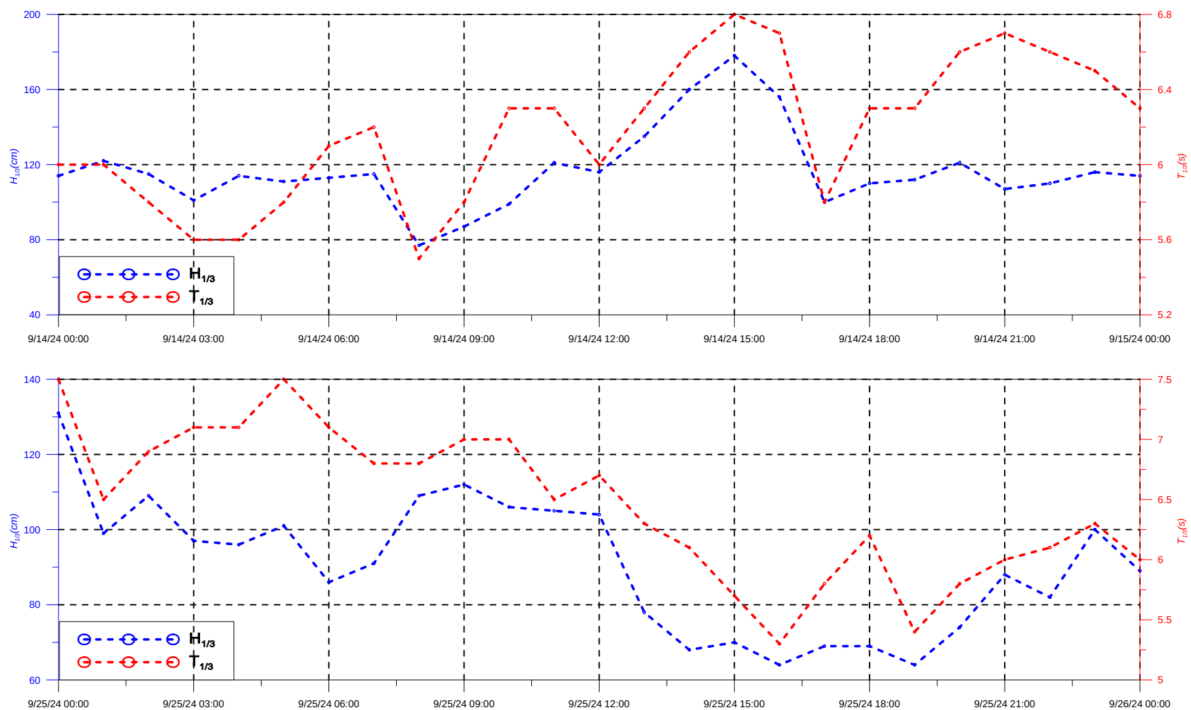
圖 2-3 波浪時序序列變化圖
