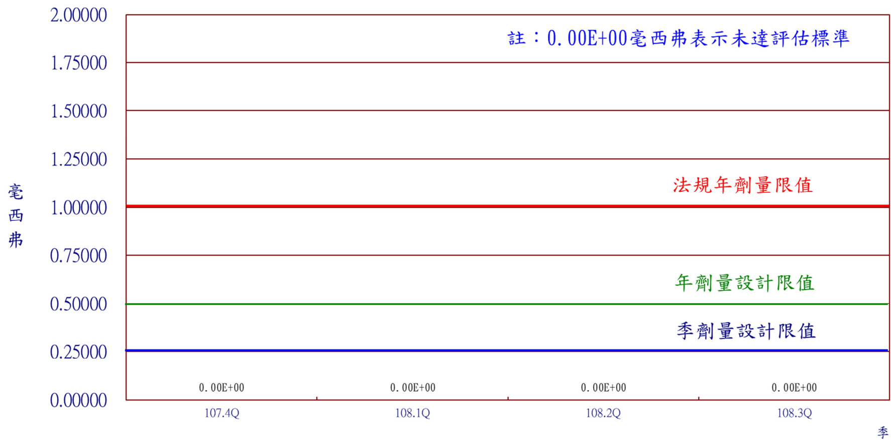
圖18 核能一廠108年第3季民眾最大個人全身劑量
