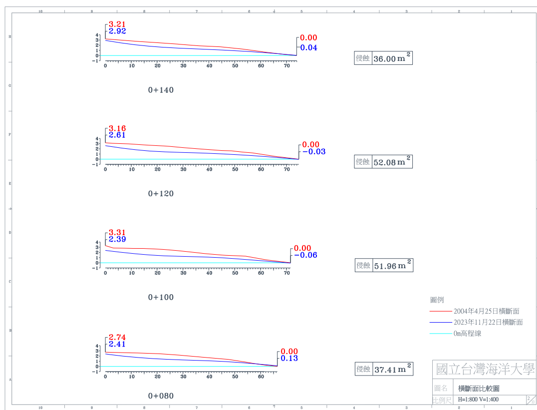
圖 4-4(i) 2023 年 11 月 22 日 A 監測區橫斷面比較圖
