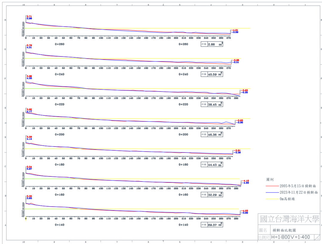
圖 4-5(e) 2023 年 11 月 22 日 B 監測區橫断面比較圖
