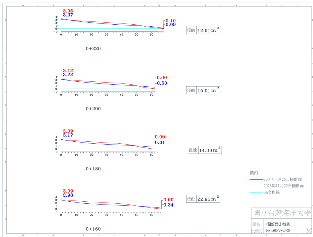
圖 4-4(h) 2023 年 11 月 22 日 A 監測區橫斷面比較圖
