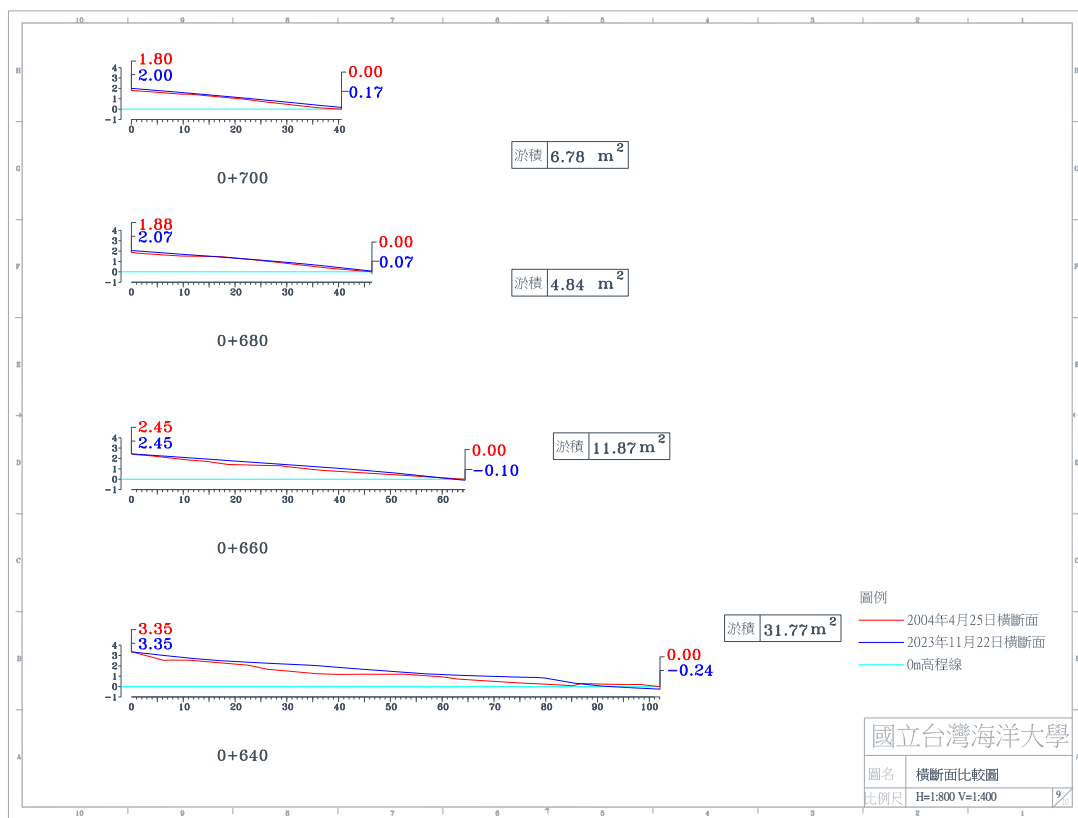
圖 4-4(b) 2023 年 11 月 22 日 A 監測區橫斷面比較圖
