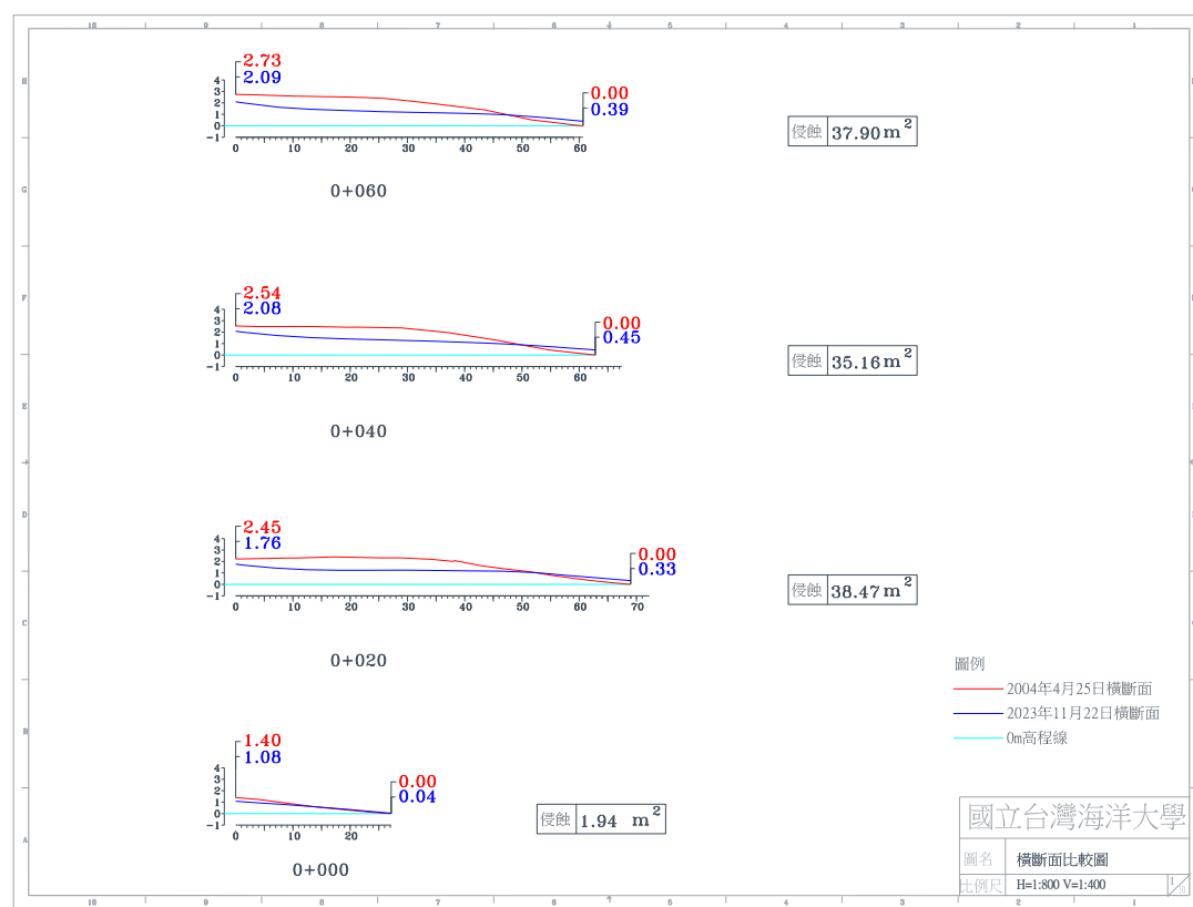
圖 4-4(j) 2023 年 11 月 22 日 A 監測區橫斷面比較圖
