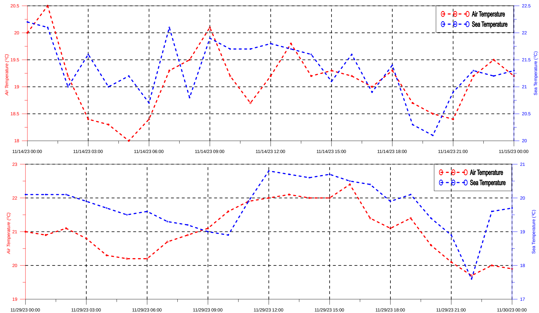
圖 2-4 溫度時序列變化圖
