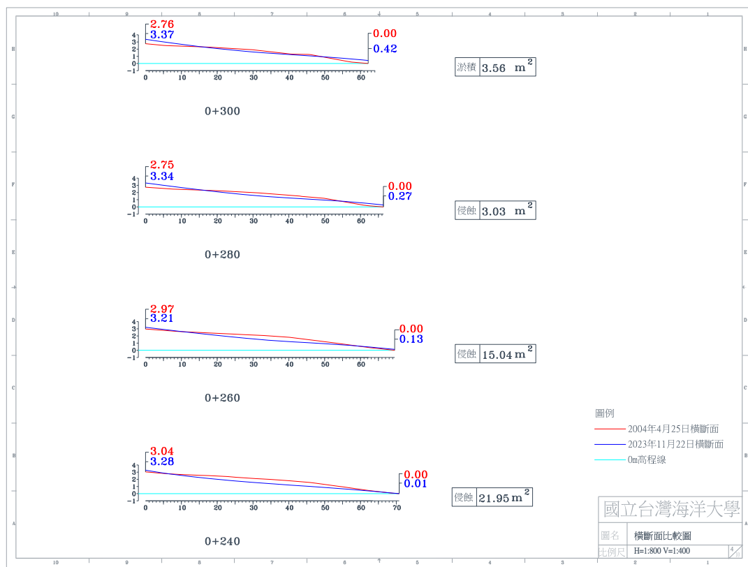
圖 4-4(g) 2023 年 11 月 22 日 A 監測區橫斷面比較圖
