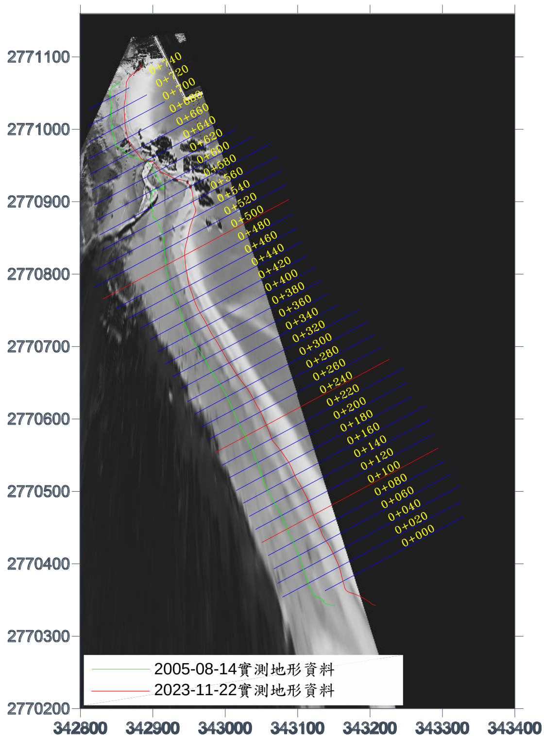
圖 4-22 長期實測 0 m 灘線比對平面示意圖(2023/11/22)
