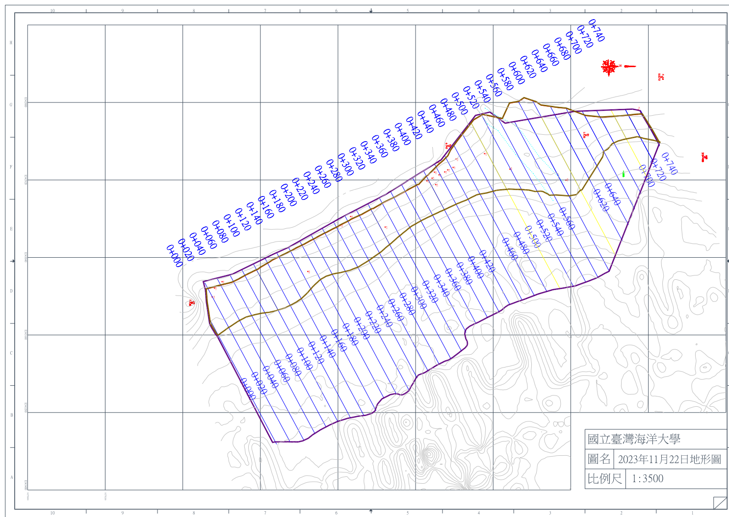
圖 4-1 2023 年 11 月 22 日監測地形
