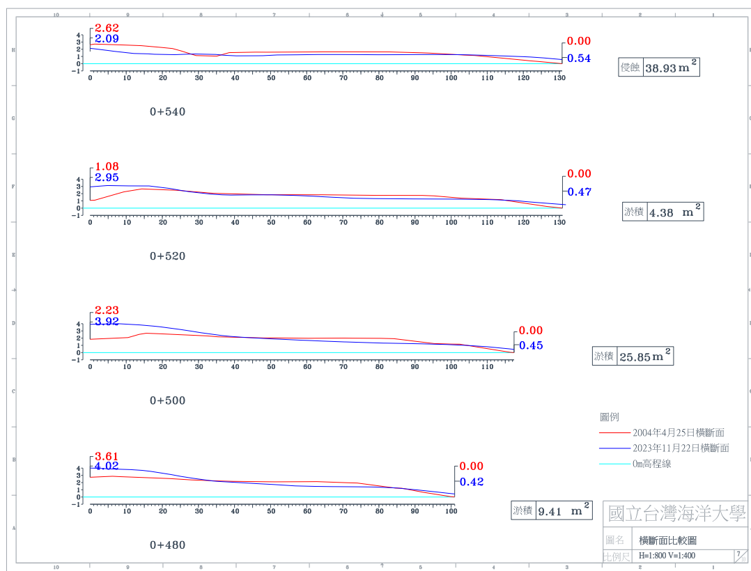
圖 4-4(d) 2023 年 11 月 22 日 A 監測區橫斷面比較圖
