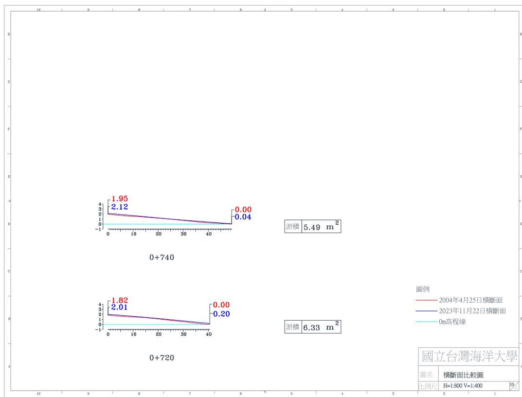
圖 4-4(a) 2023 年 11 月 22 日 A 監測區橫斷面比較圖
