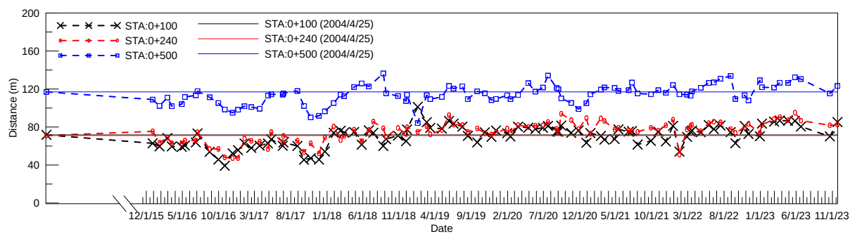
圖 4-21 岸線斷面沙灘寬度變化圖(2023/11/22)
