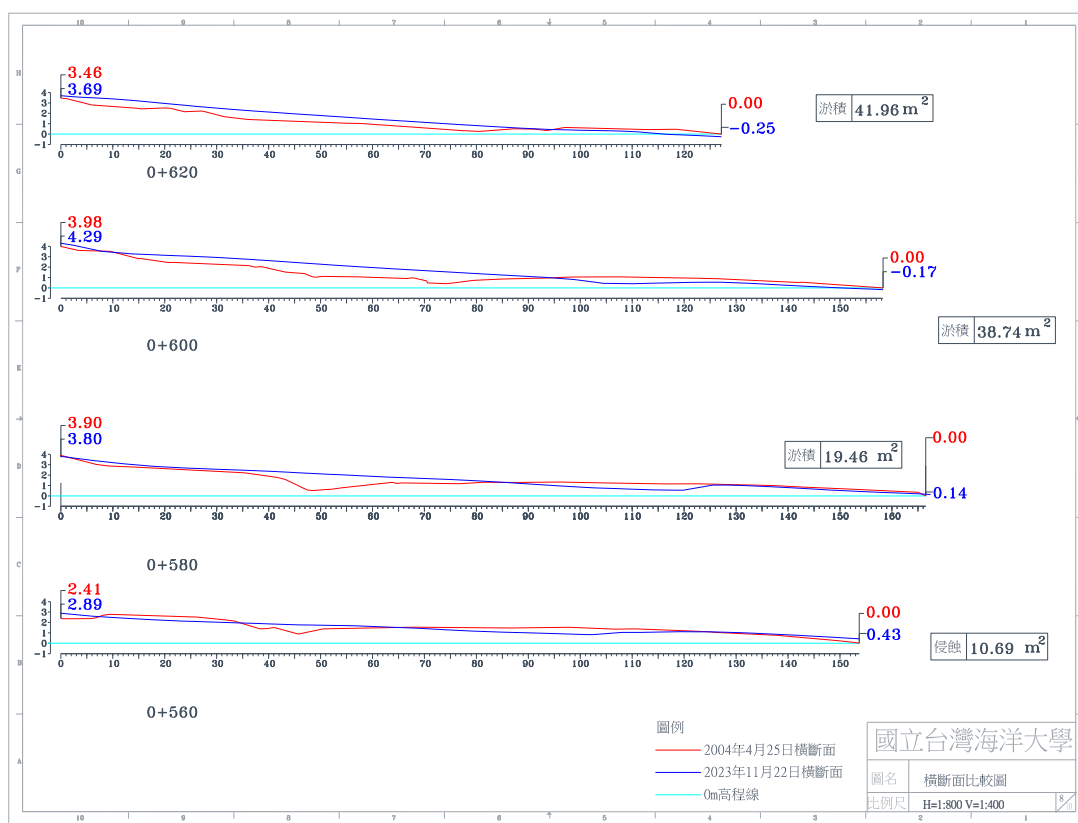
圖 4-4(c) 2023 年 11 月 22 日 A 監測區橫斷面比較圖
