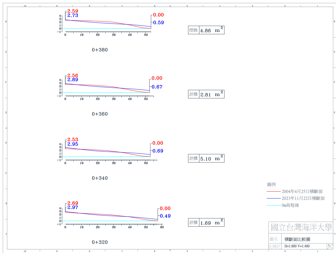
圖 4-4(f) 2023 年 11 月 22 日 A 監測區橫斷面比較圖
