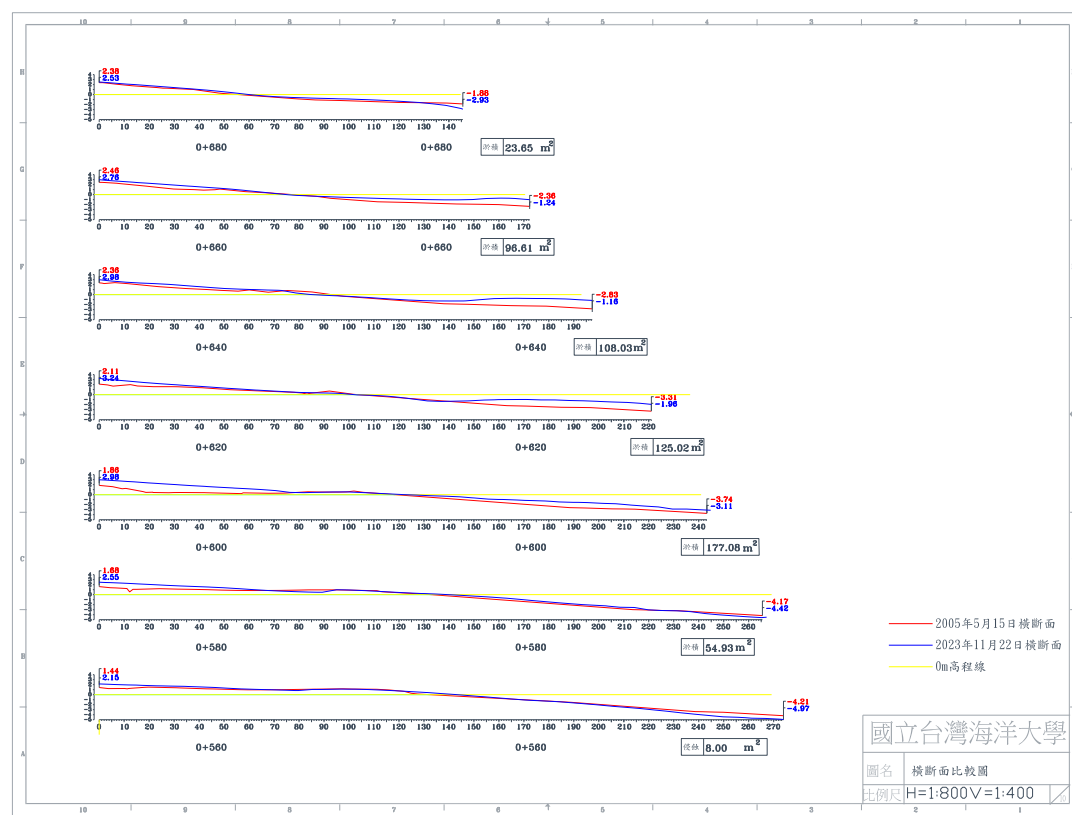
圖 4-5(b) 2023 年 11 月 22 日 B 監測區橫斷面比較圖
