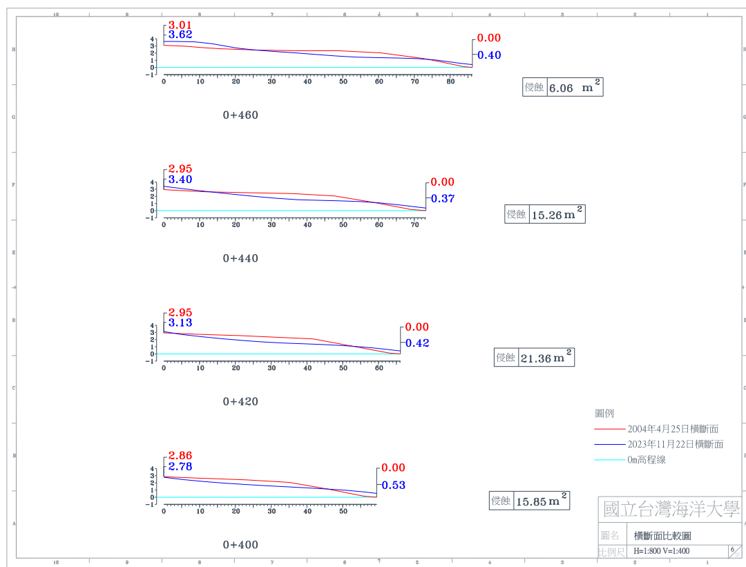
圖 4-4(e) 2023 年 11 月 22 日 A 監測區橫斷面比較圖
