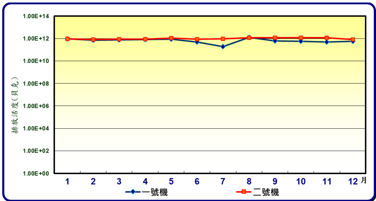
圖 7 113 年各廢氣排放源總排放活度統計圖
