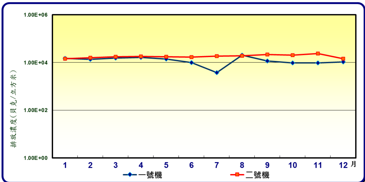
圖 8 113 年各廢氣排放源總排放濃度統計圖
