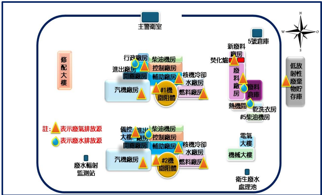
圖 1 放射性廢氣、廢水排放源位置圖
