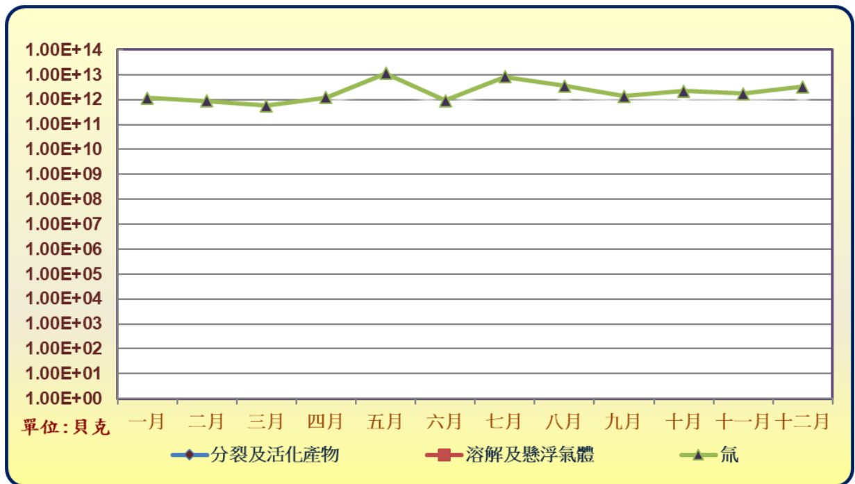
圖 9 113 年放射性廢水排放活度統計圖
