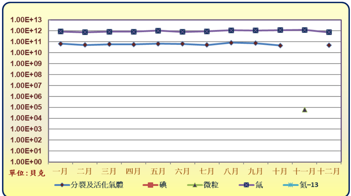
圖 6 113 年二號機放射性廢氣排放活度統計圖
