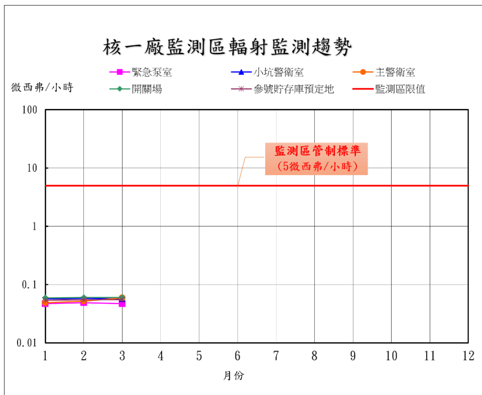
圖 4 監測區輻射監測趨勢
