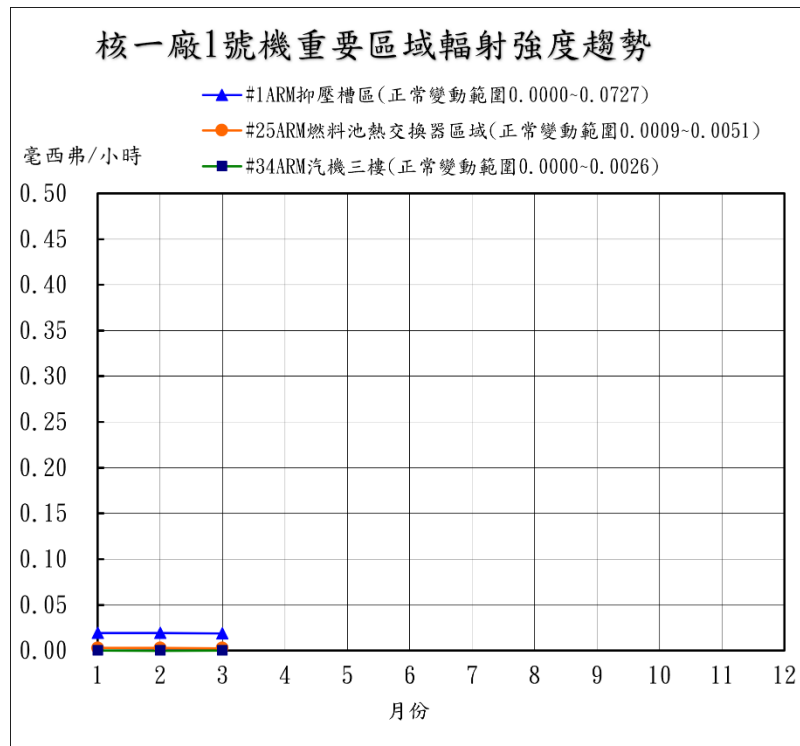
圖 1 核一廠 1 號機重要區域輻射強度趨勢
