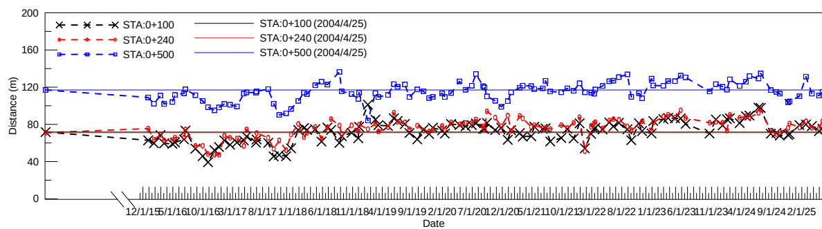
圖 4-21 岸線斷面沙灘寬度變化圖(2025/05/17)
