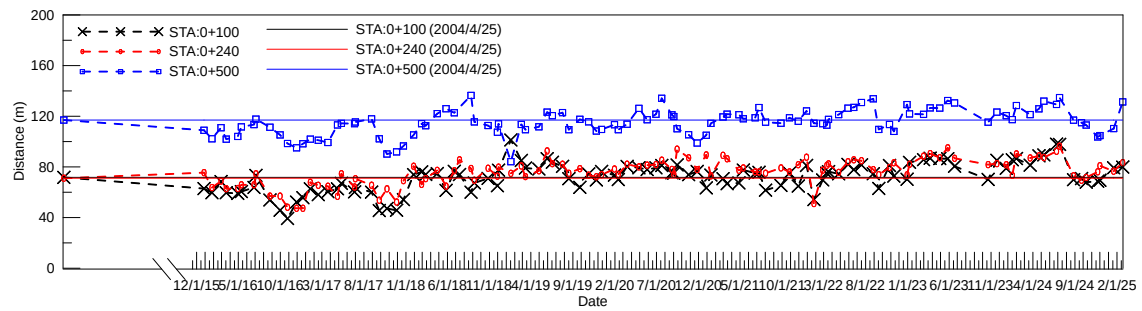
圖 4-16 岸線斷面沙灘寬度變化圖(2025/02/22)
