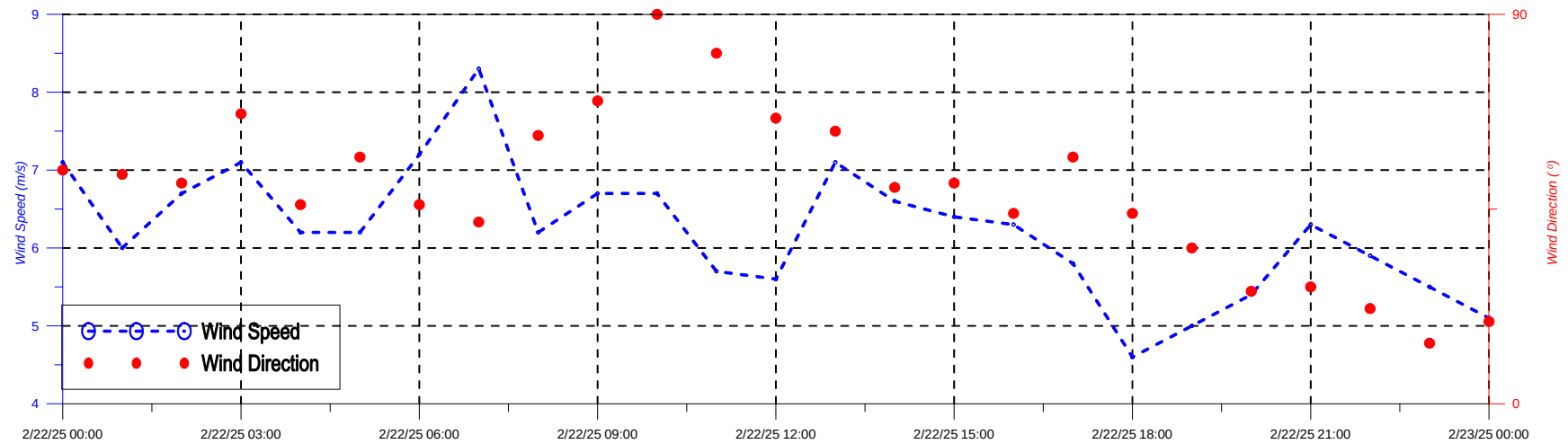
圖 2-2 風速風向時序序列變化圖
