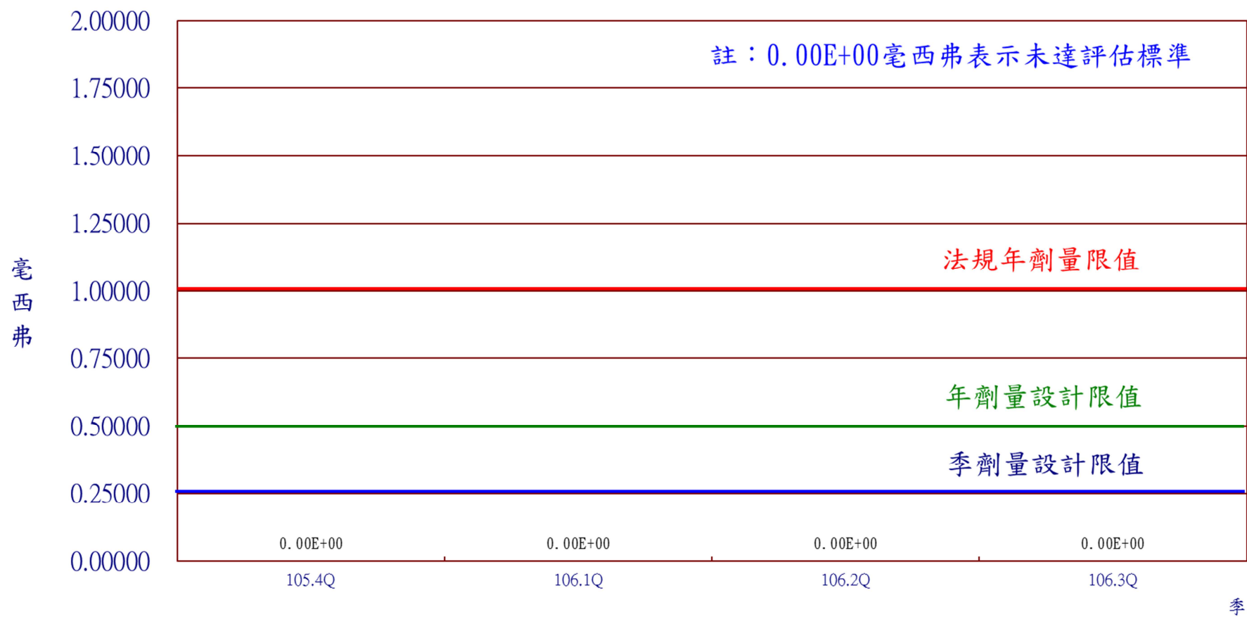
圖18 核能一廠106年第3季民眾最大個人全身劑量
