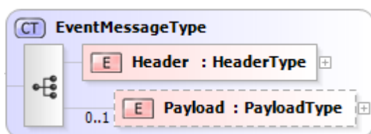
圖 3-7 created(EndDeviceEvents).EventMessageType 訊息格式
