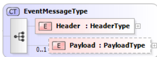
圖 3-3 created(MeterReadings).EventMessageType 訊息格式
