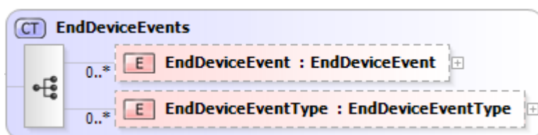
圖 3-8 created(EndDeviceEvents).EventMessageType.Payload.EndDeviceEvents 訊息格式
