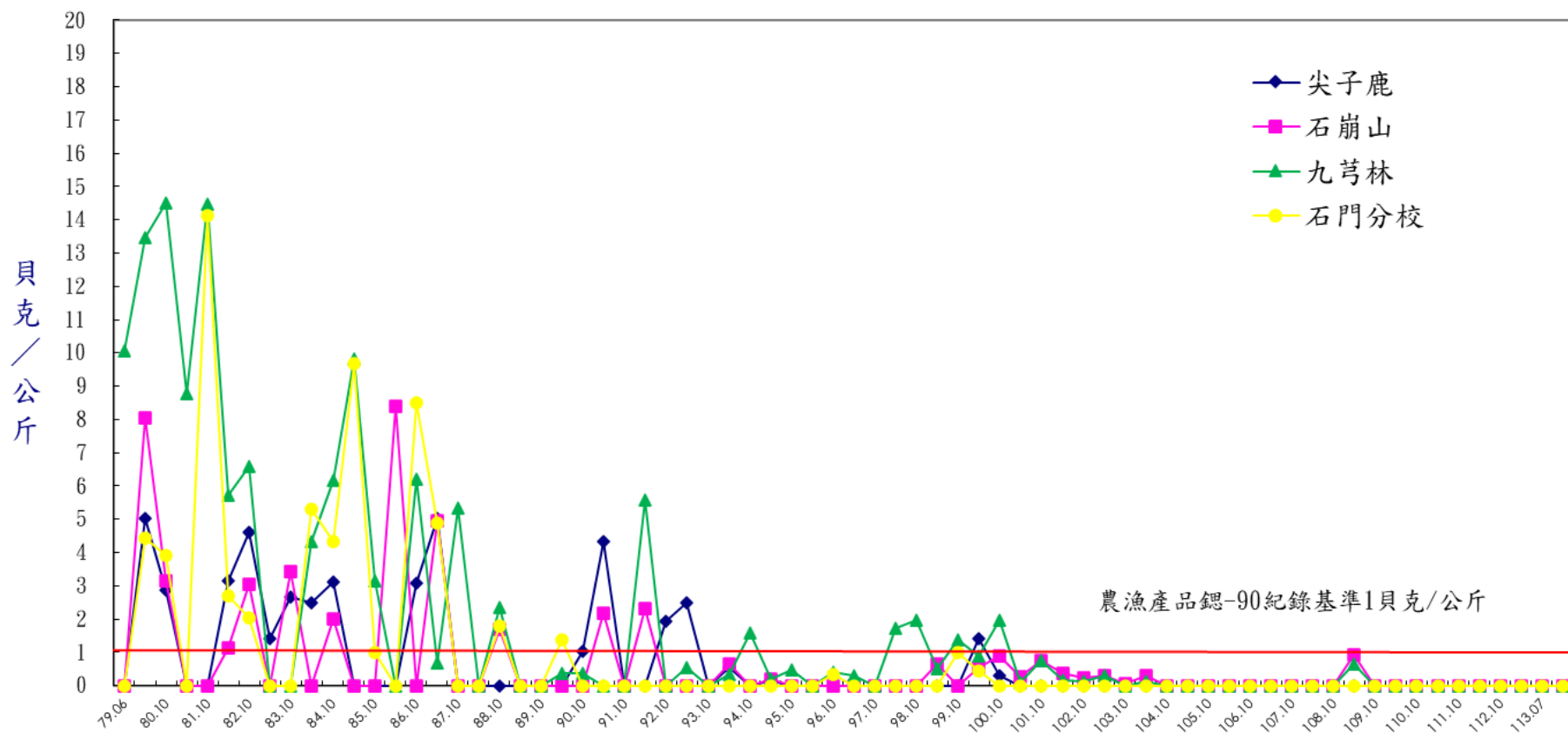
圖16 核能一廠茶葉銨-90活度歷年分析結果
