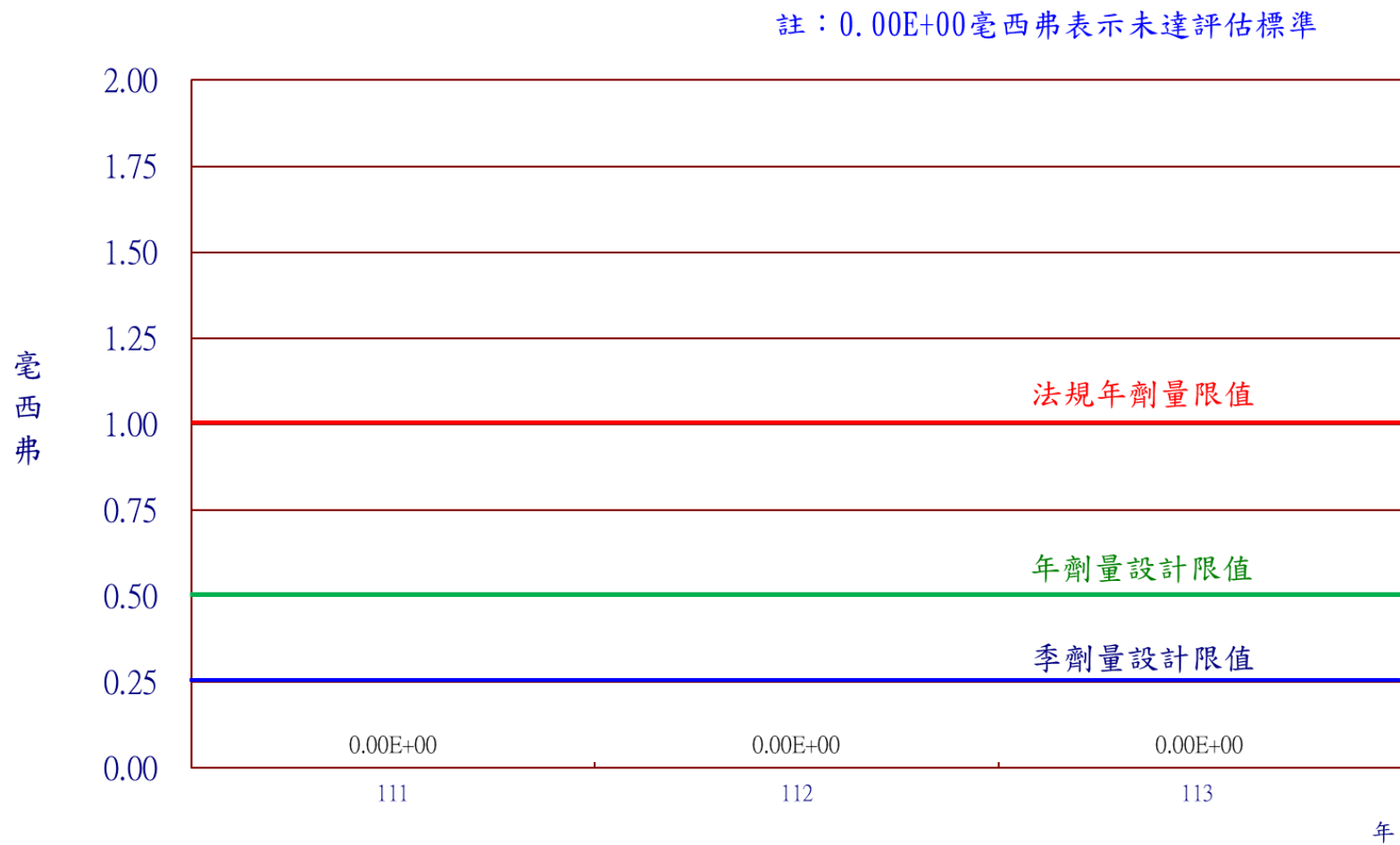
圖18 核能一廠113年民眾最大個人全身劑量
