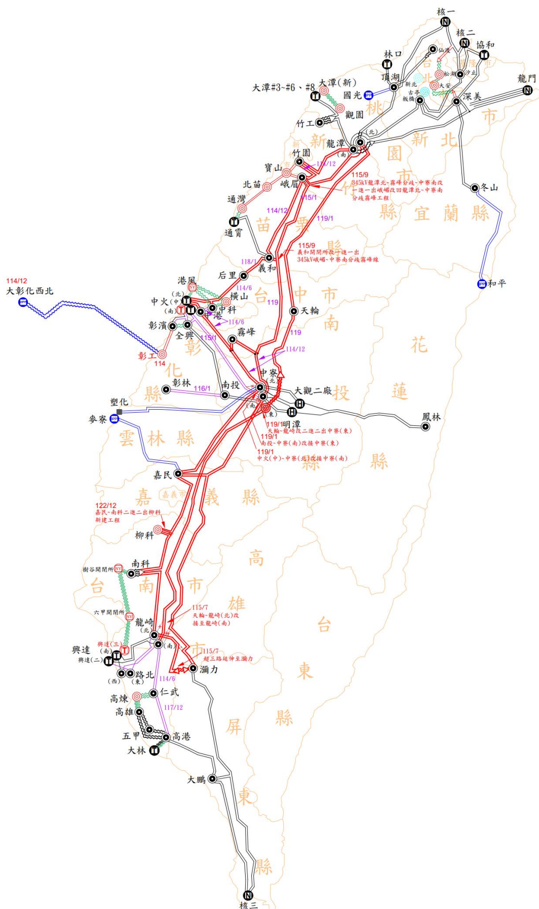
附圖 超高壓主幹線系統圖(粗線)
