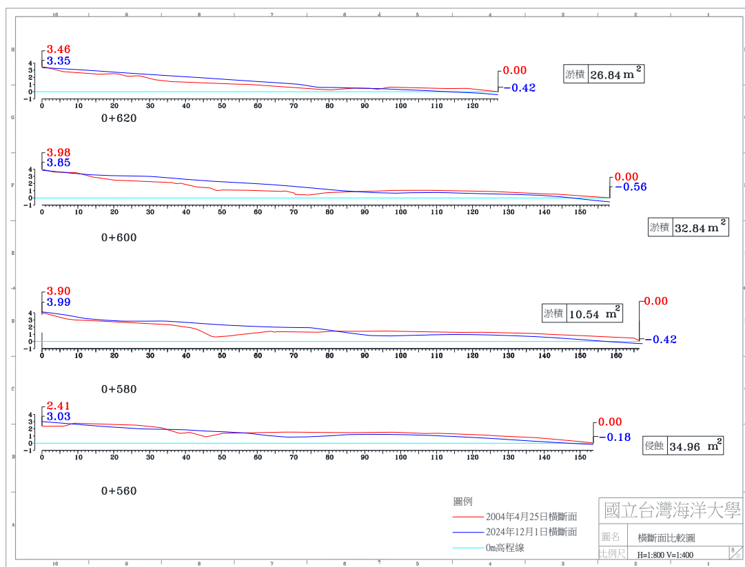
圖 4-4(c) 2024 年 12 月 1 日 A 監測區橫斷面比較圖
