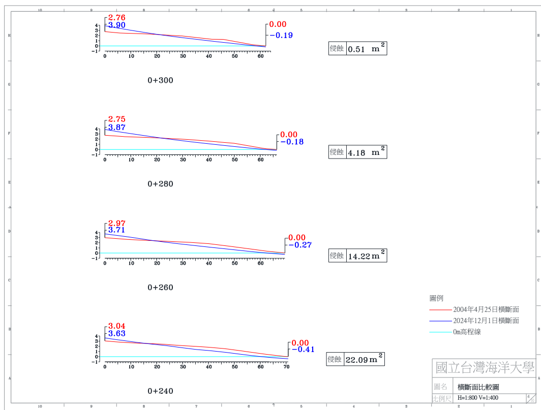
圖 4-4(g) 2024 年 12 月 1 日 A 監測區橫斷面比較圖
