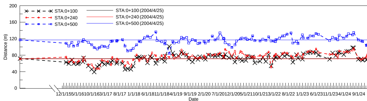
圖 4-21 岸線斷面沙灘寬度變化圖(2024/12/01)
