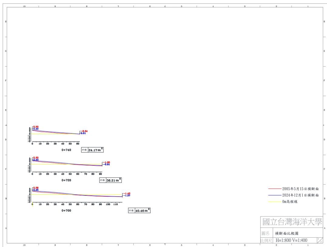
圖 4-5(a) 2024 年 12 月 1 日 B 監測區橫斷面比較圖
