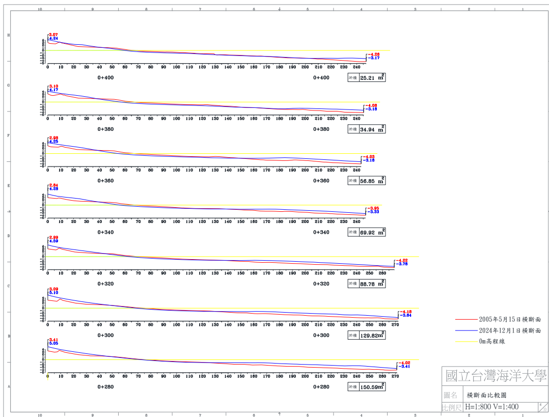
圖 4-5(d) 2024 年 12 月 1 日 B 監測區橫断面比較圖
