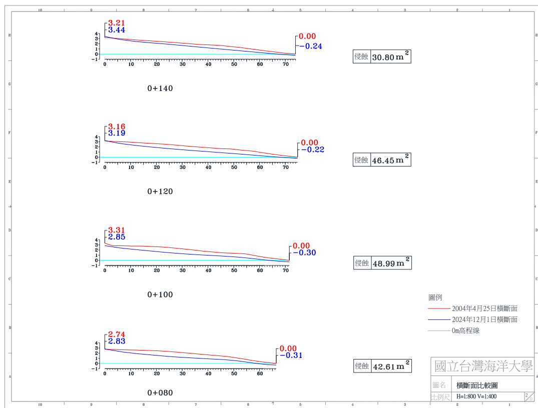
圖 4-4(i) 2024 年 12 月 1 日 A 監測區橫斷面比較圖
