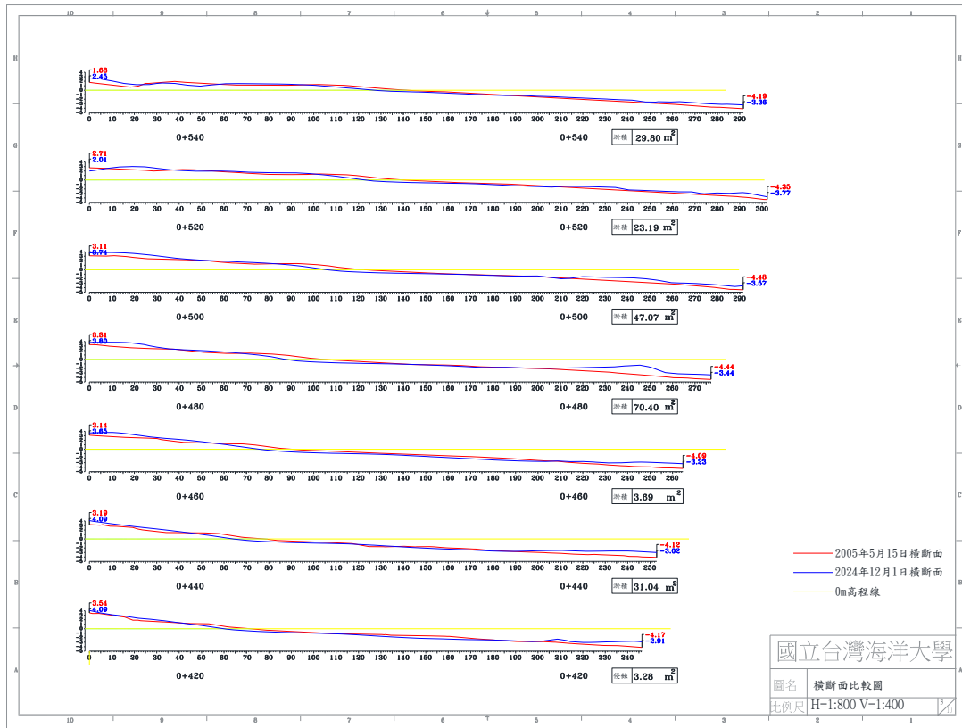
圖 4-5(c) 2024 年 12 月 1 日 B 監測區橫断面比較圖
