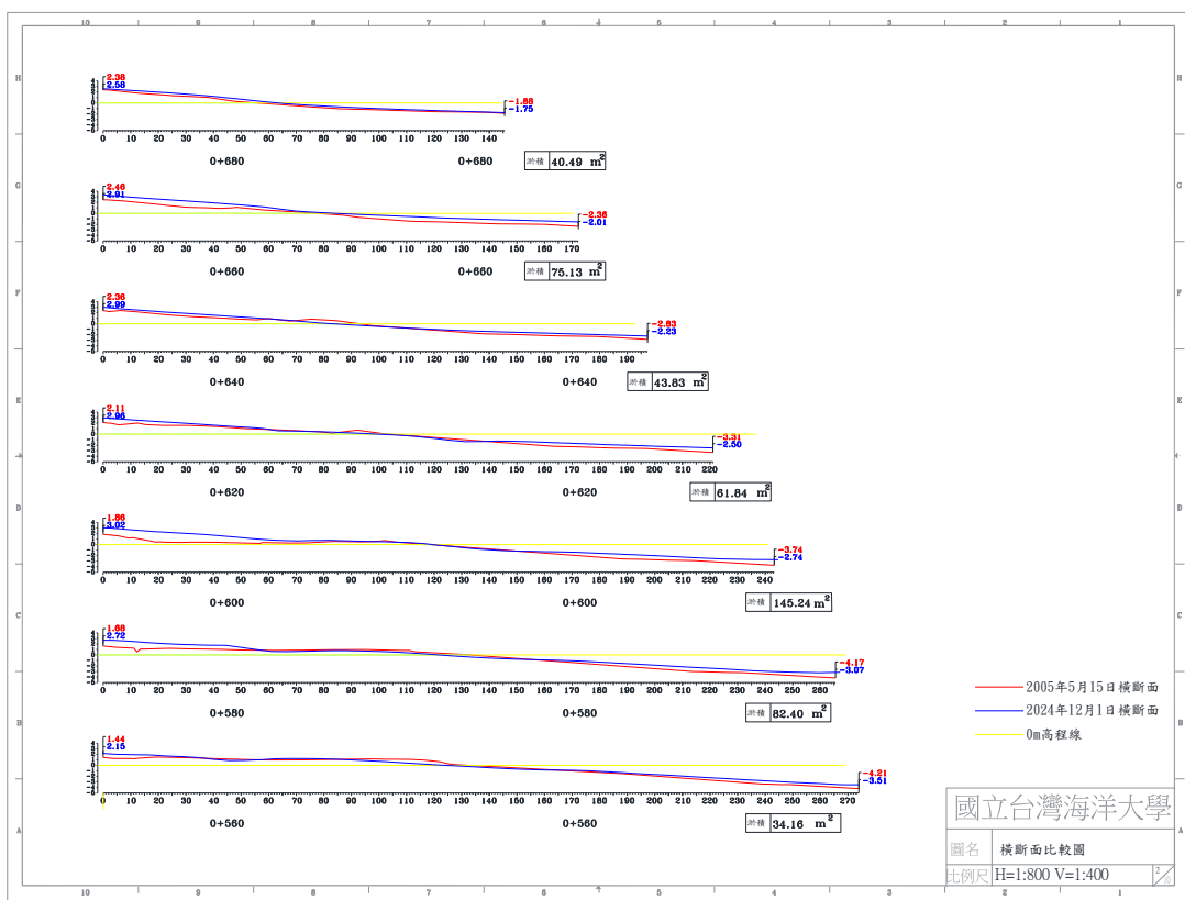
圖 4-5(b) 2024 年 12 月 1 日 B 監測區橫斷面比較圖
