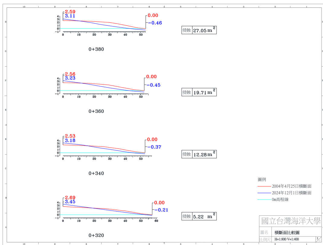
圖 4-4(f) 2024 年 12 月 1 日 A 監測區橫斷面比較圖
