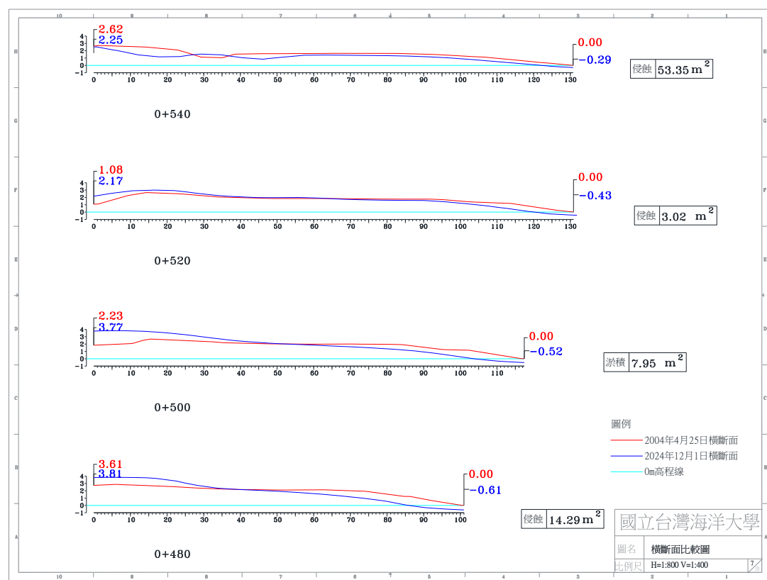
圖 4-4(d) 2024 年 12 月 1 日 A 監測區橫斷面比較圖
