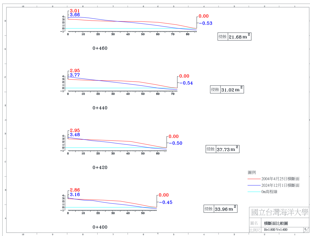
圖 4-4(e) 2024 年 12 月 1 日 A 監測區橫斷面比較圖
