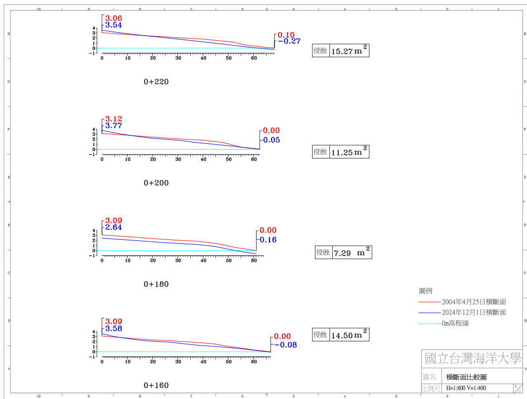
圖 4-4(h) 2024 年 12 月 1 日 A 監測區橫斷面比較圖
