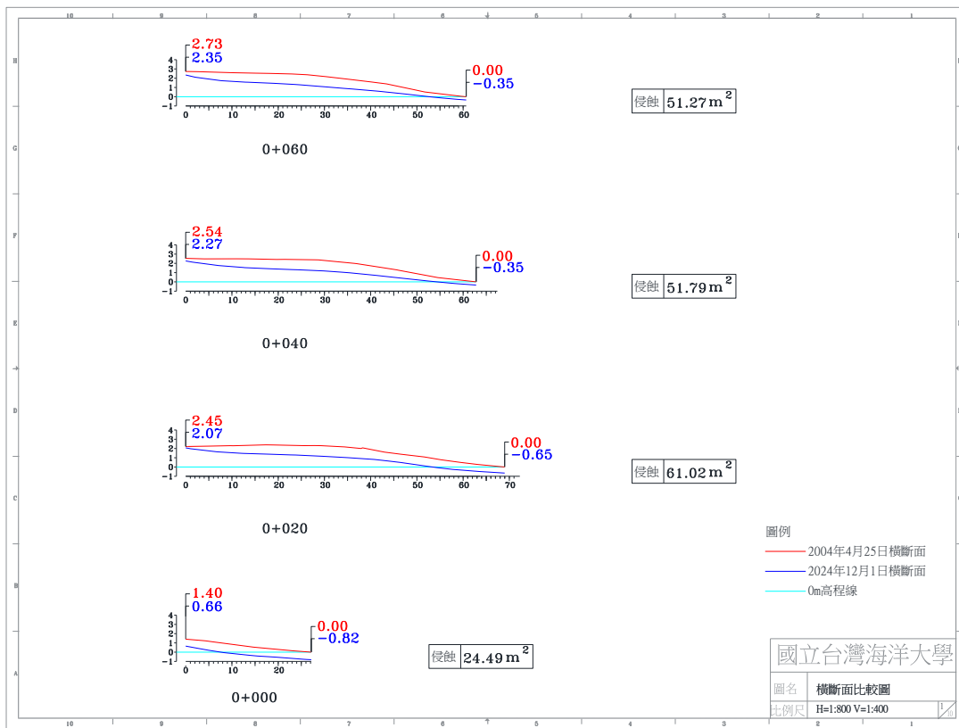
圖 4-4(j) 2024 年 12 月 1 日 A 監測區橫斷面比較圖
