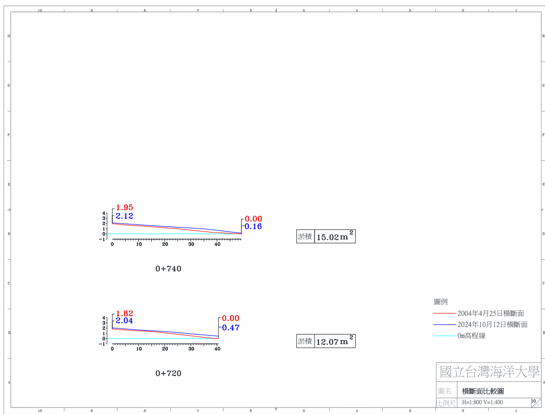
圖 4-4(a) 2024 年 10 月 12 日 A 監測區橫斷面比較圖
