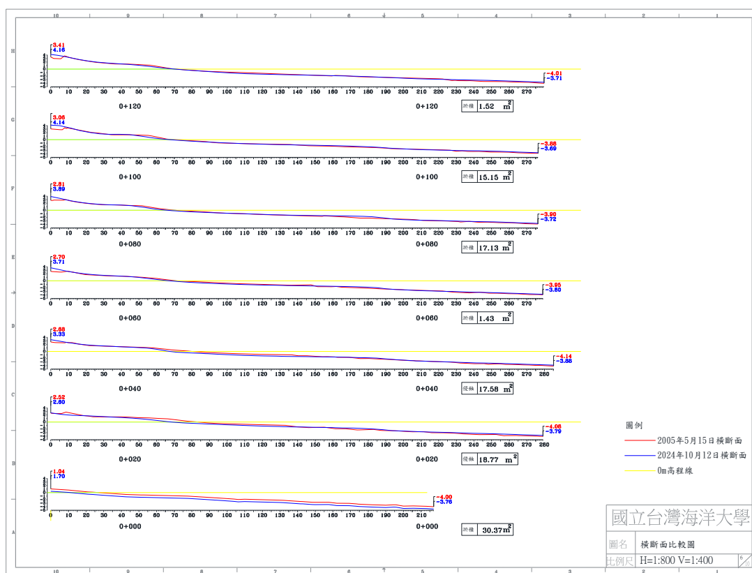
圖 4-5(f) 2024 年 10 月 12 日 B 監測區橫断面比較圖
