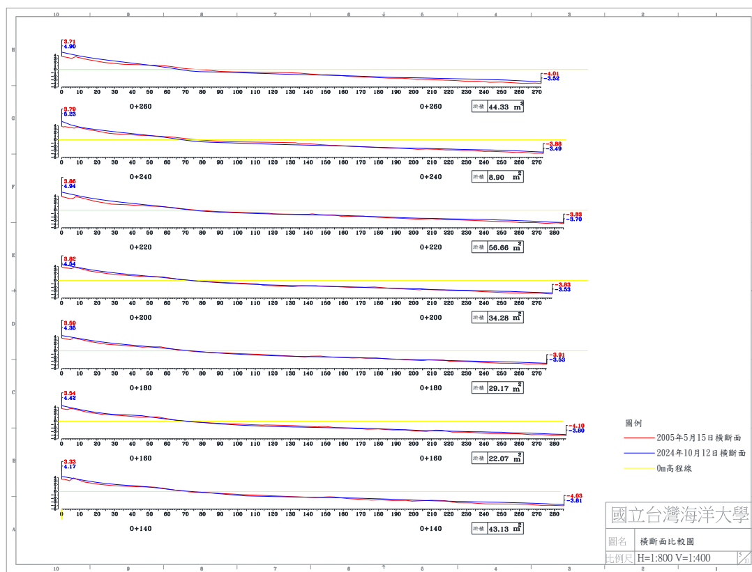
圖 4-5(e) 2024 年 10 月 12 日 B 監測區橫断面比較圖
