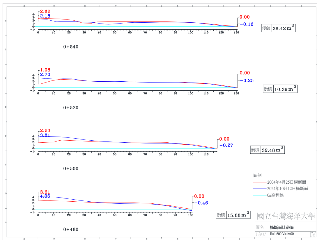
圖 4-4(d) 2024 年 10 月 12 日 A 監測區橫斷面比較圖
