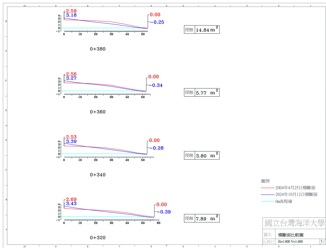
圖 4-4(f) 2024 年 10 月 12 日 A 監測區橫斷面比較圖
