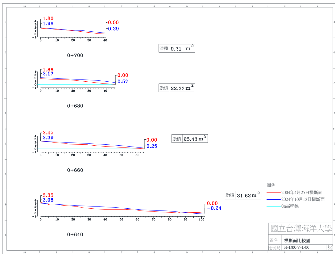
圖 4-4(b) 2024 年 10 月 12 日 A 監測區橫斷面比較圖
