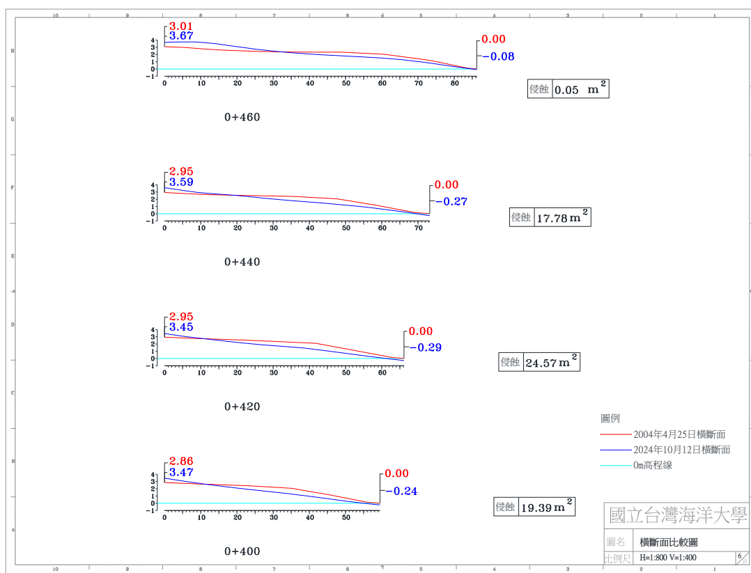
圖 4-4(e) 2024 年 10 月 12 日 A 監測區橫斷面比較圖
