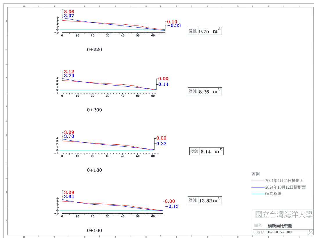
圖 4-4(h) 2024 年 10 月 12 日 A 監測區橫斷面比較圖
