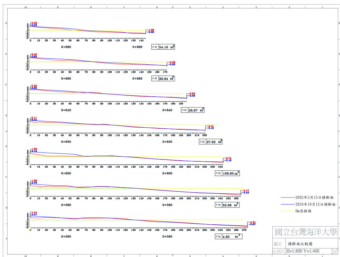
圖 4-5(b) 2024 年 10 月 12 日 B 監測區橫斷面比較圖
