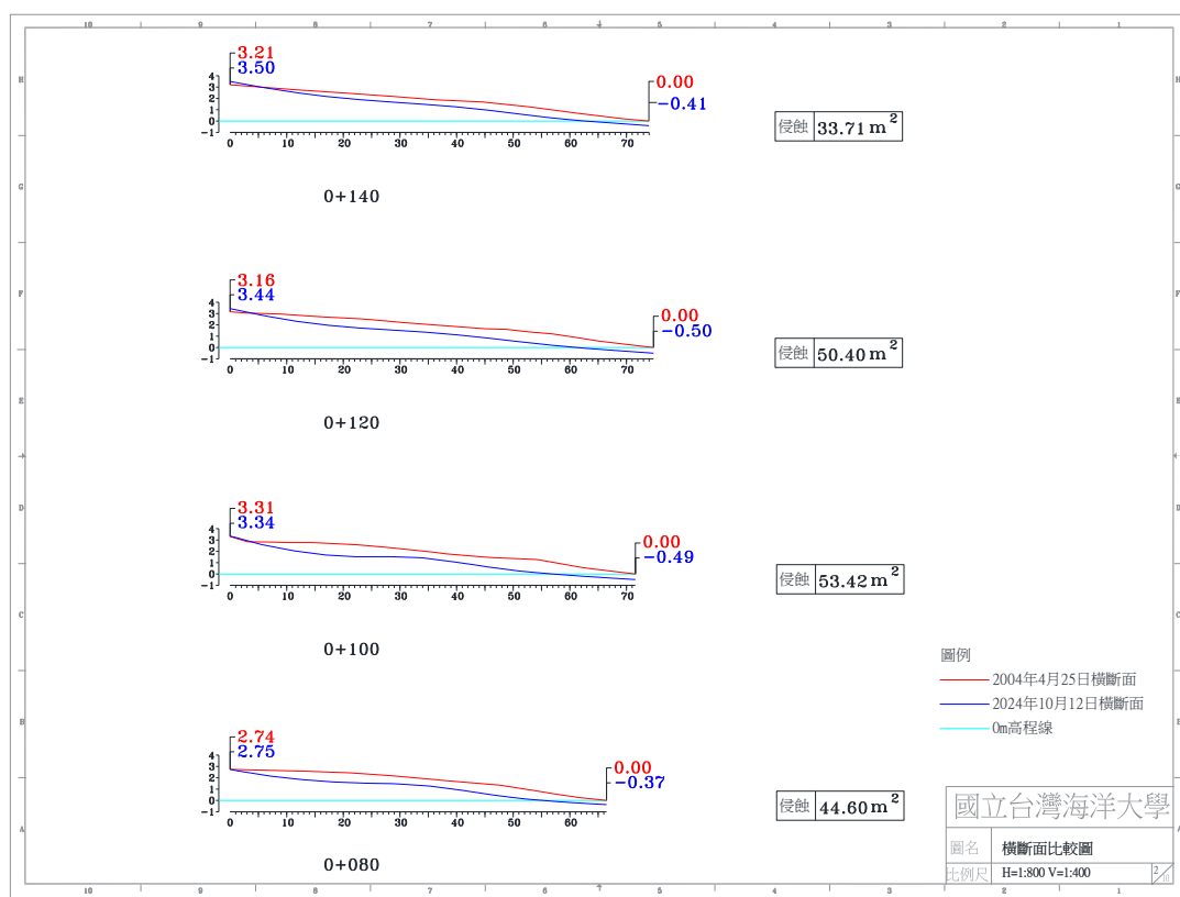
圖 4-4(i) 2024 年 10 月 12 日 A 監測區橫斷面比較圖
