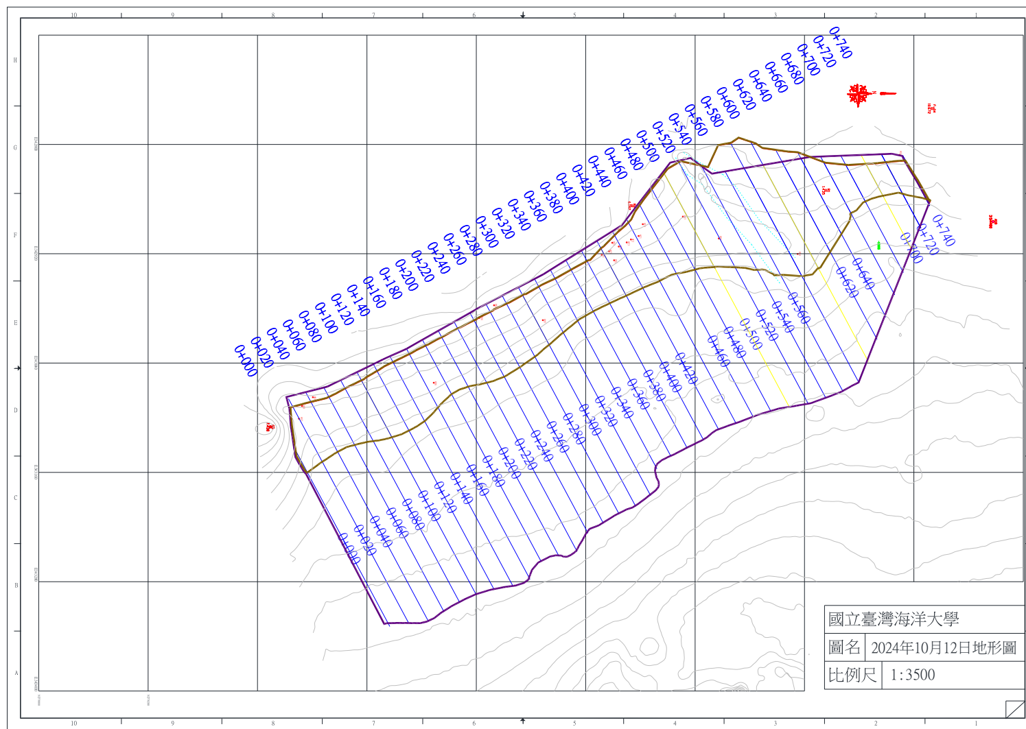
圖 4-1 2024 年 10 月 12 日監測地形
