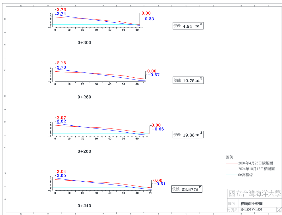
圖 4-4(g) 2024 年 10 月 12 日 A 監測區橫斷面比較圖
