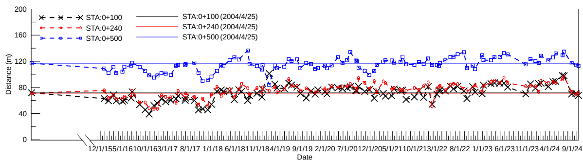
圖 4-21 岸線斷面沙灘寬度變化圖(2024/10/12)
