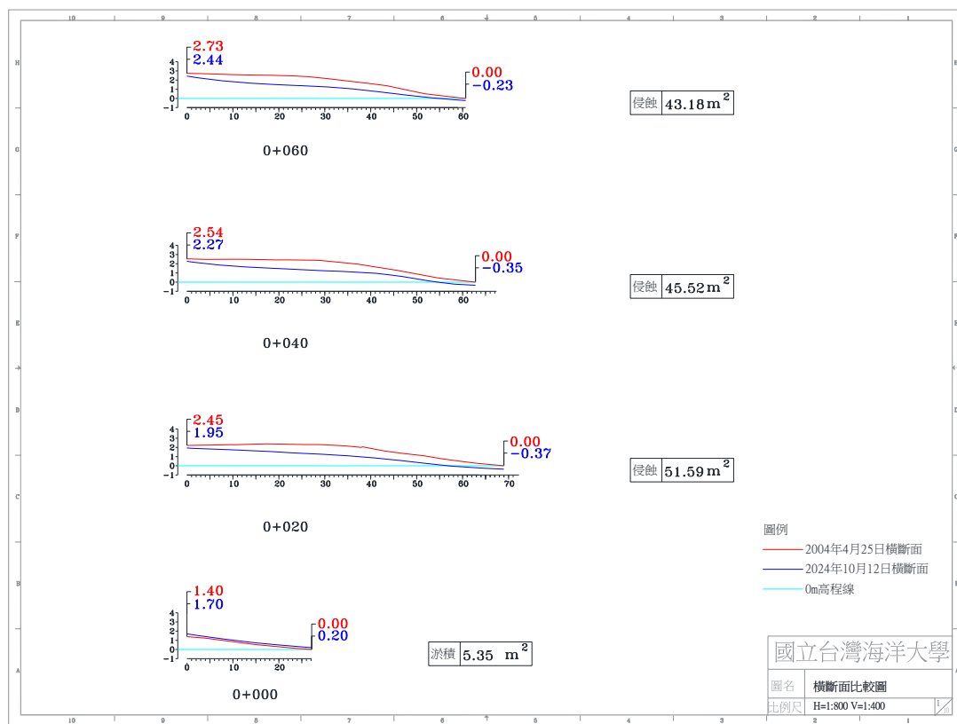
圖 4-4(j) 2024 年 10 月 12 日 A 監測區橫斷面比較圖
