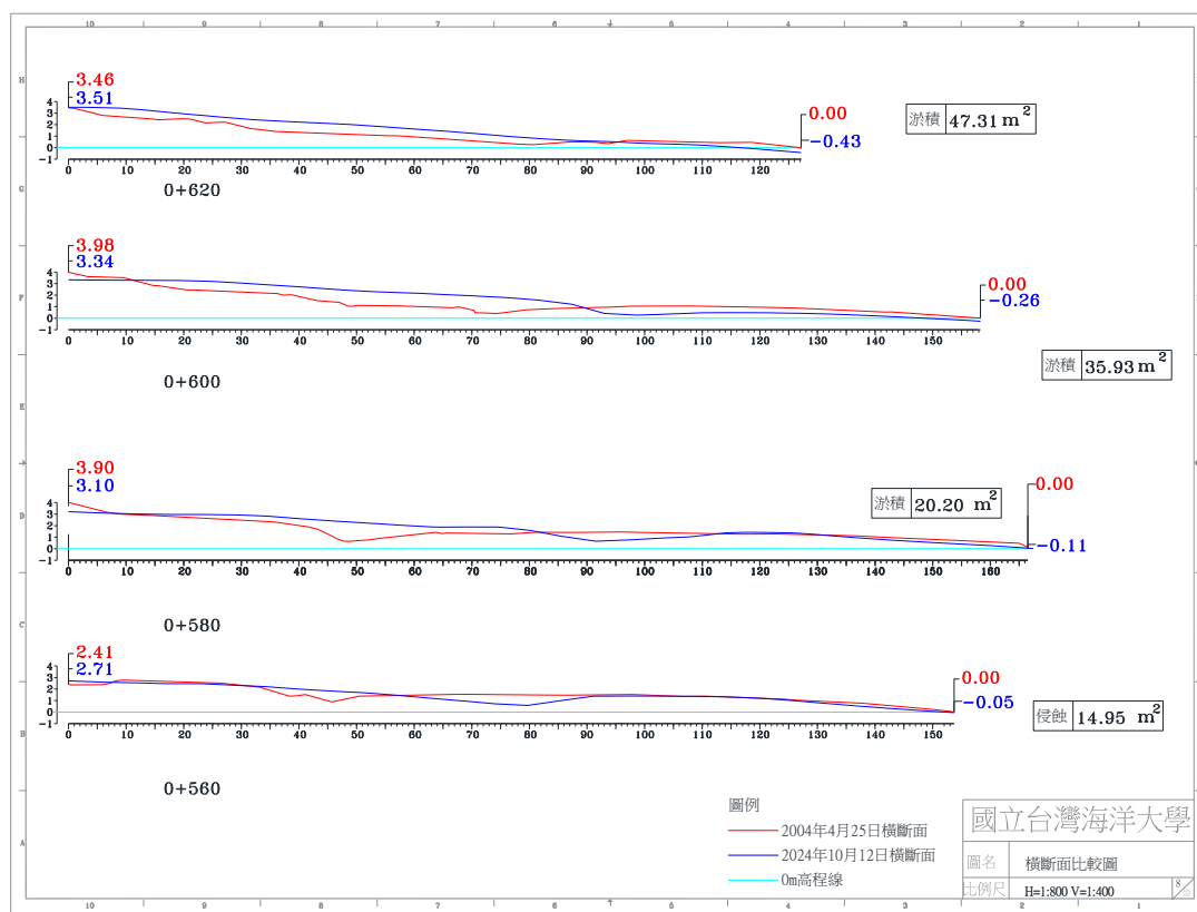
圖 4-4(c) 2024 年 10 月 12 日 A 監測區橫斷面比較圖
