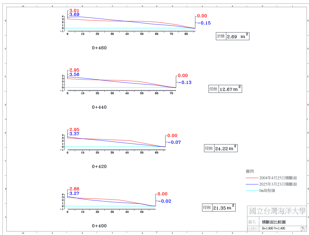
圖 4-4(e) 2025 年 3 月 23 日 A 監測區橫斷面比較圖
