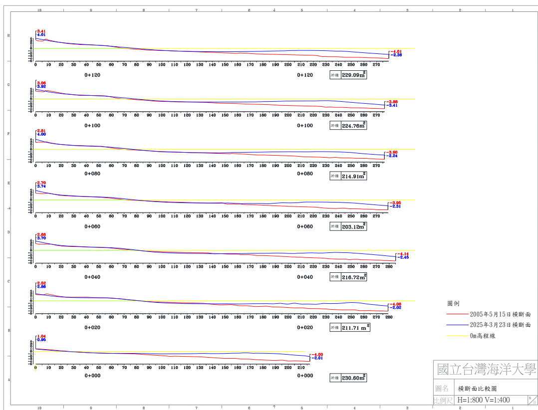
圖 4-5(f) 2025 年 3 月 23 日 B 監測區橫断面比較圖
