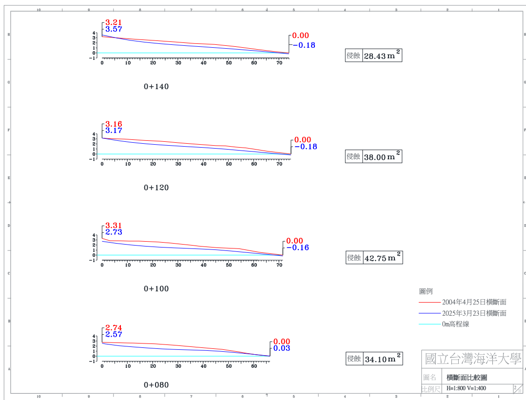
圖 4-4(i) 2025 年 3 月 23 日 A 監測區橫斷面比較圖
