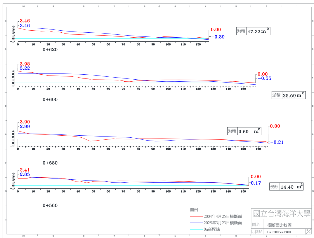
圖 4-4(c) 2025 年 3 月 23 日 A 監測區橫斷面比較圖
