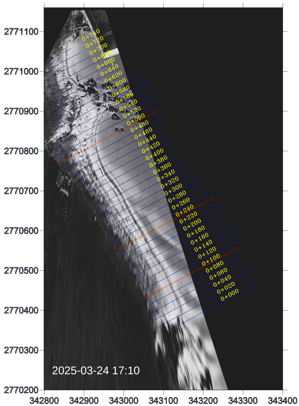
圖 4-19 鹽寮海岸地形影像全景圖(2025/03/24 17:10)
