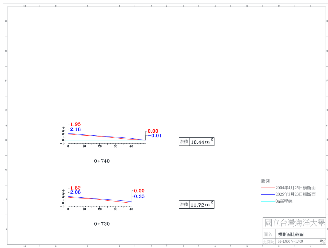
圖 4-4(a) 2025 年 3 月 23 日 A 監測區橫斷面比較圖
