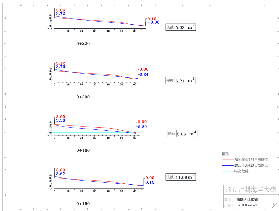
圖 4-4(h) 2025 年 3 月 23 日 A 監測區橫斷面比較圖
