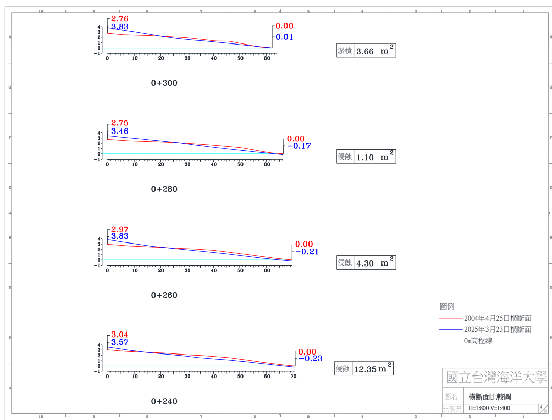
圖 4-4(g) 2025 年 3 月 23 日 A 監測區橫斷面比較圖
