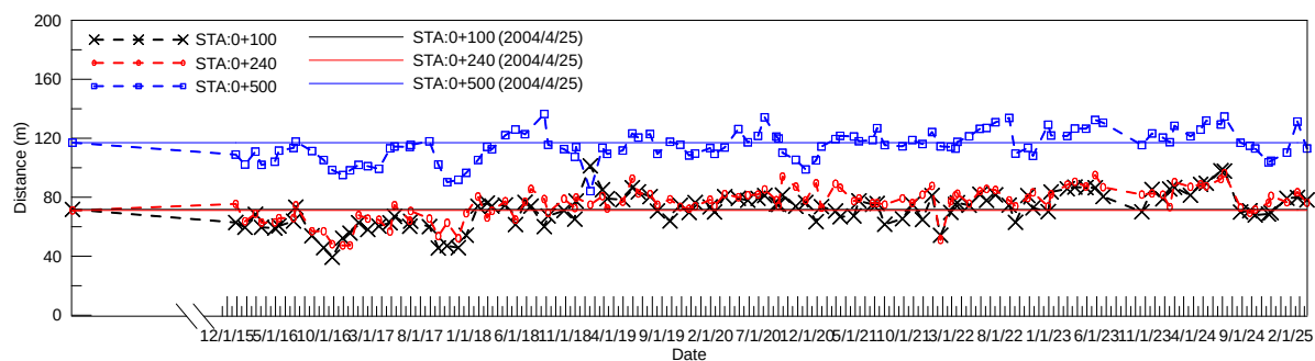
圖 4-21 岸線斷面沙灘寬度變化圖(2025/03/24)
