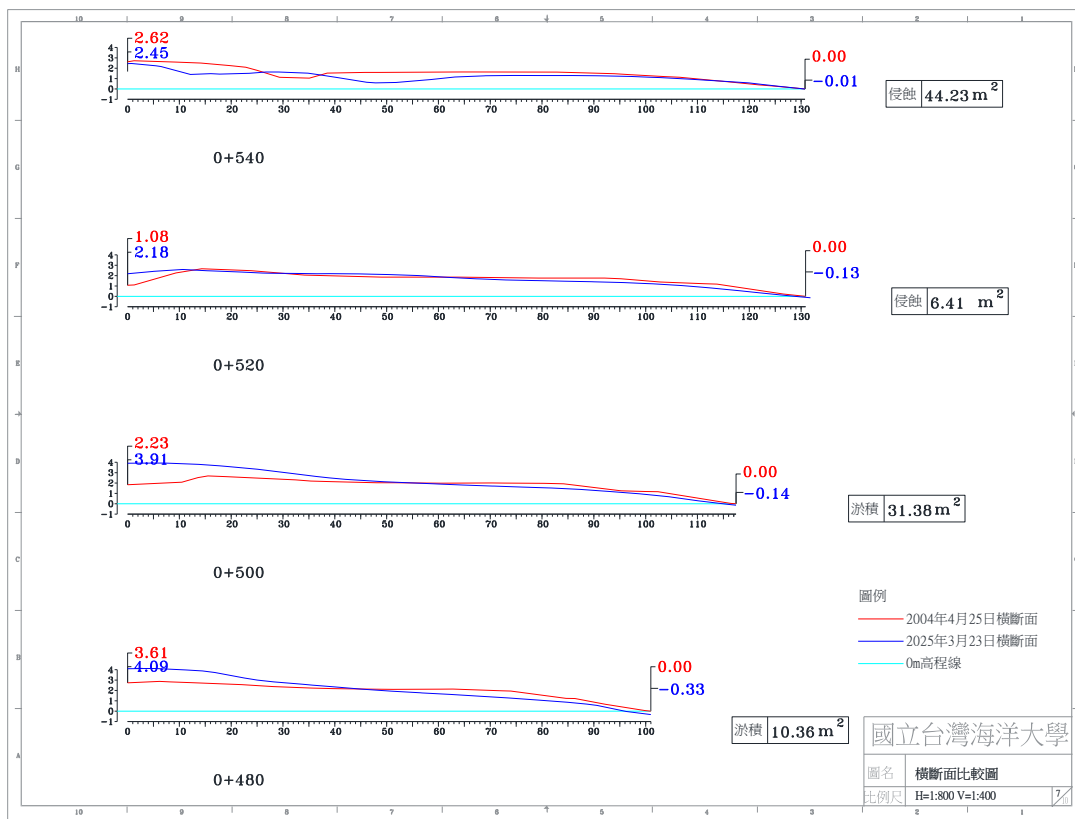
圖 4-4(d) 2025 年 3 月 23 日 A 監測區橫斷面比較圖
