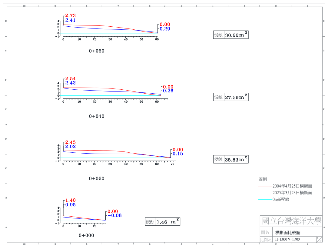
圖 4-4(j) 2025 年 3 月 23 日 A 監測區橫斷面比較圖
