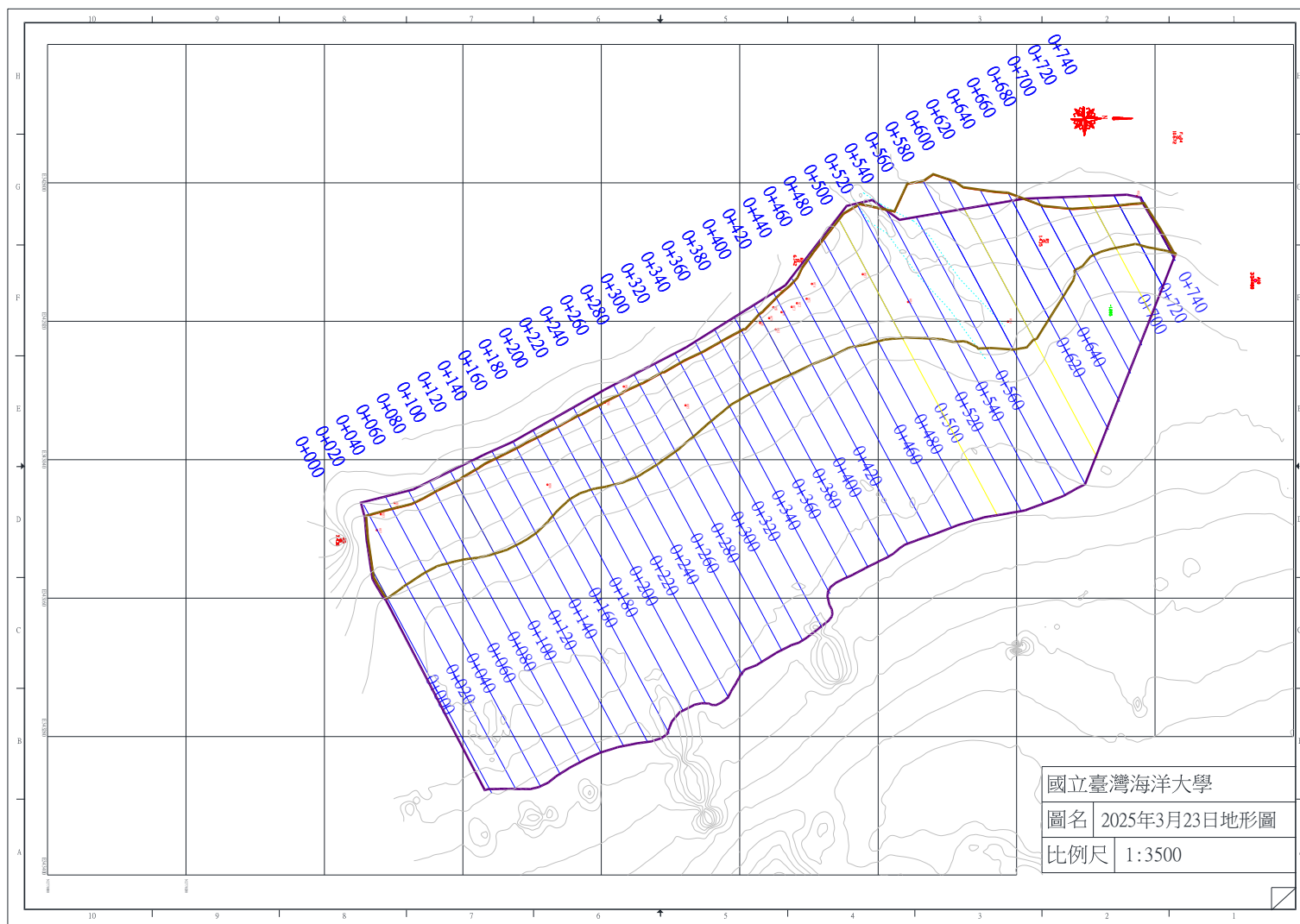
圖 4-1 2025 年 3 月 23 日監測地形
