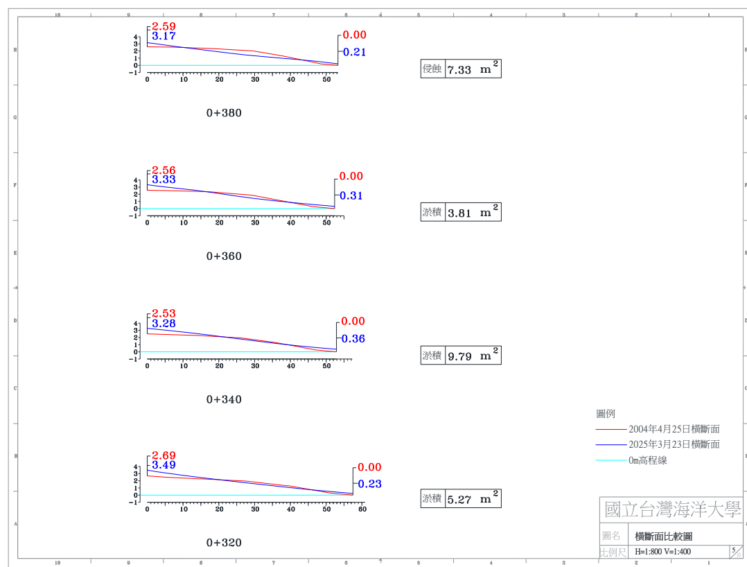
圖 4-4(f) 2025 年 3 月 23 日 A 監測區橫斷面比較圖
