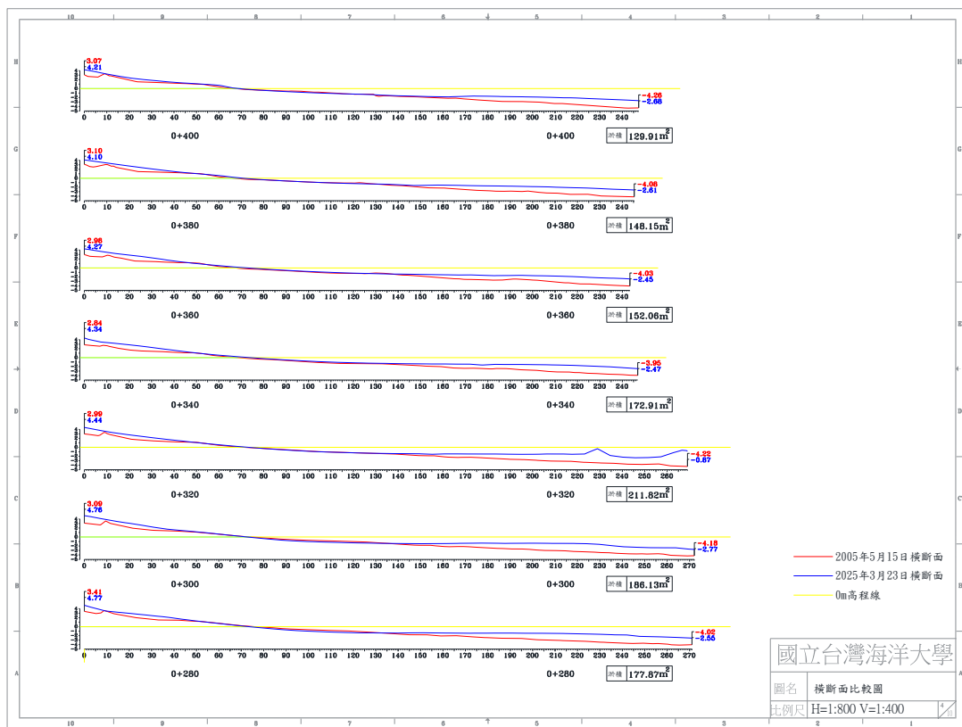
圖 4-5(d) 2025 年 3 月 23 日 B 監測區橫斷面比較圖
