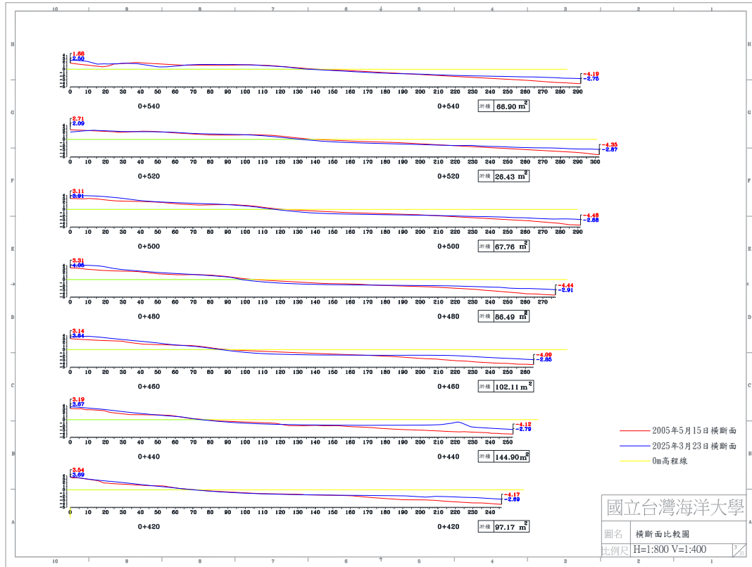
圖 4-5(c) 2025 年 3 月 23 日 B 監測區橫斷面比較圖
