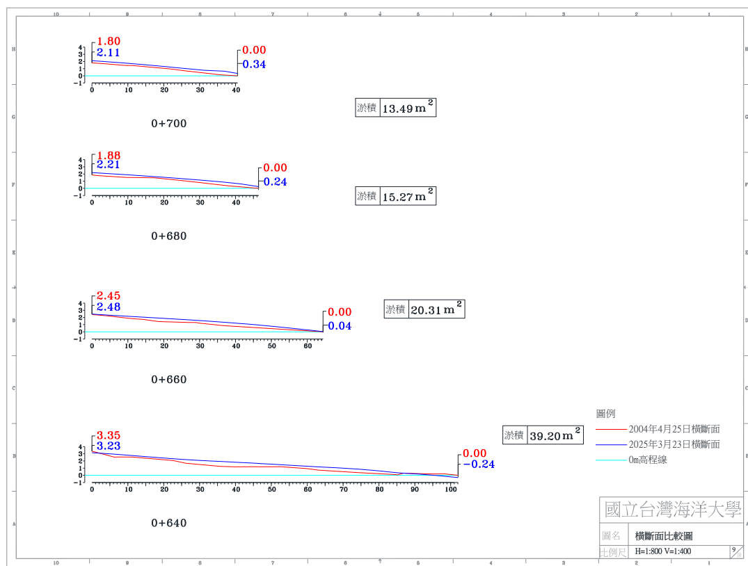
圖 4-4(b) 2025 年 3 月 23 日 A 監測區橫斷面比較圖
