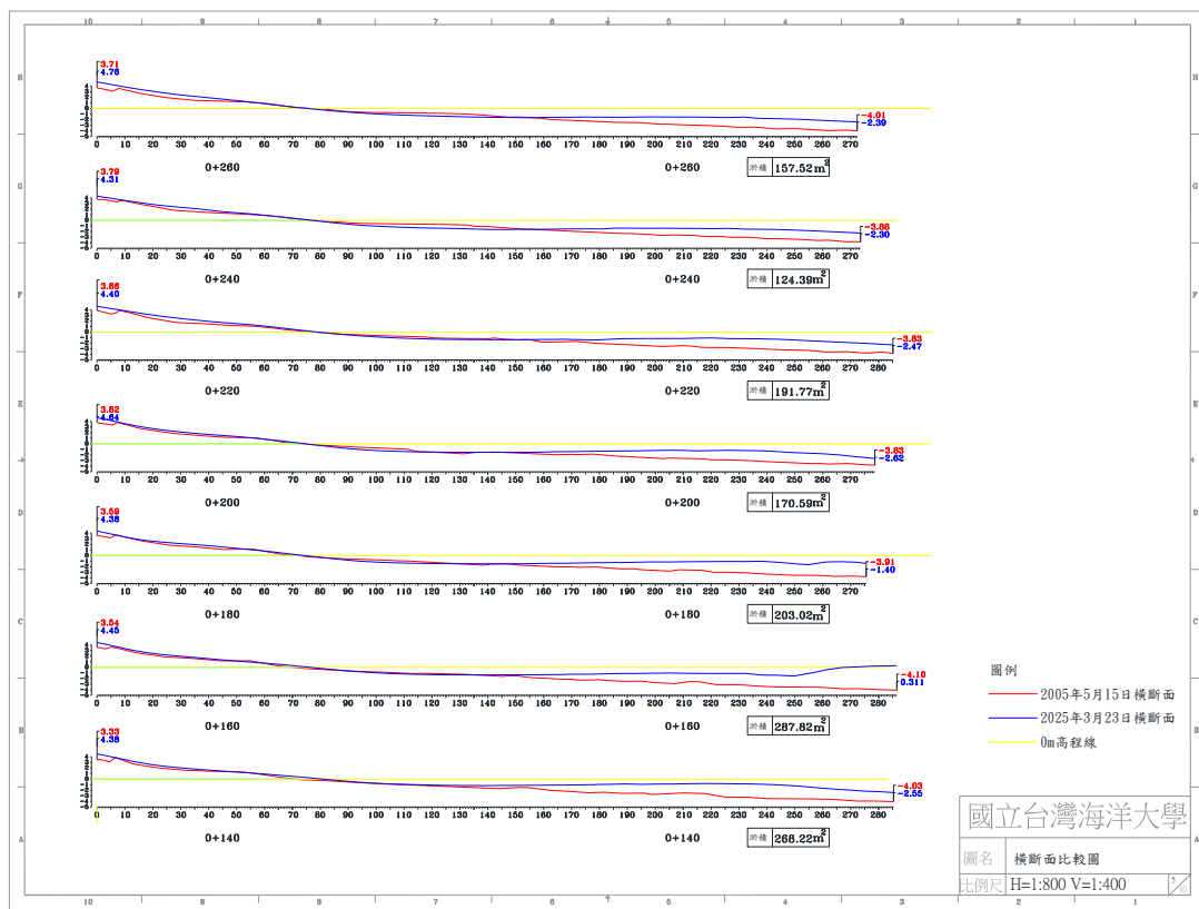
圖 4-5(e) 2025 年 3 月 23 日 B 監測區橫断面比較圖
