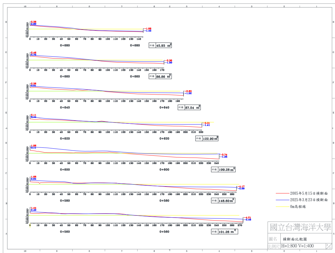
圖 4-5(b) 2025 年 3 月 23 日 B 監測區橫斷面比較圖
