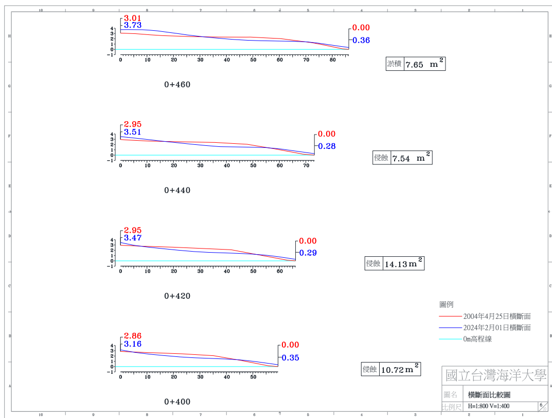
圖 4-4(e) 2024 年 2 月 1 日 A 監測區橫斷面比較圖
