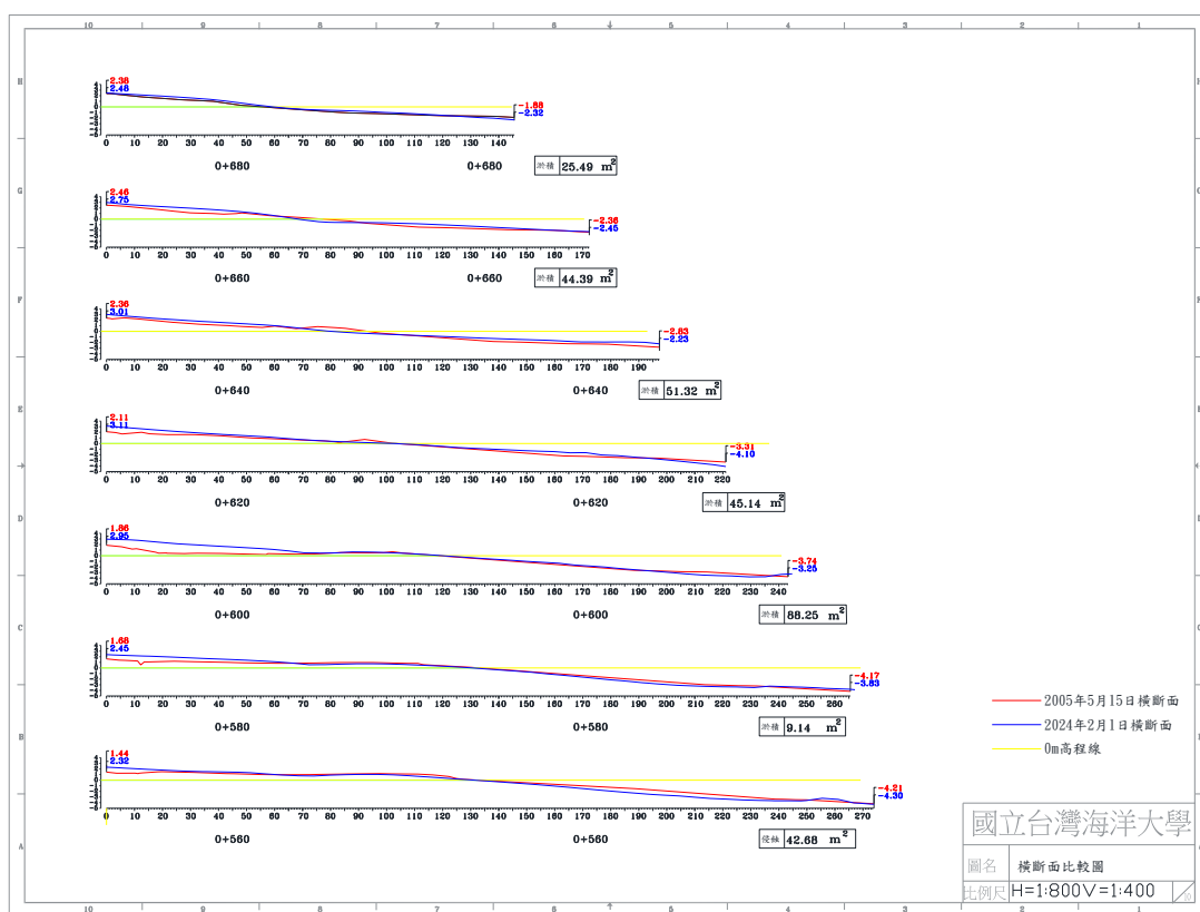
圖 4-5(b) 2024 年 2 月 1 日 B 監測區橫斷面比較圖
