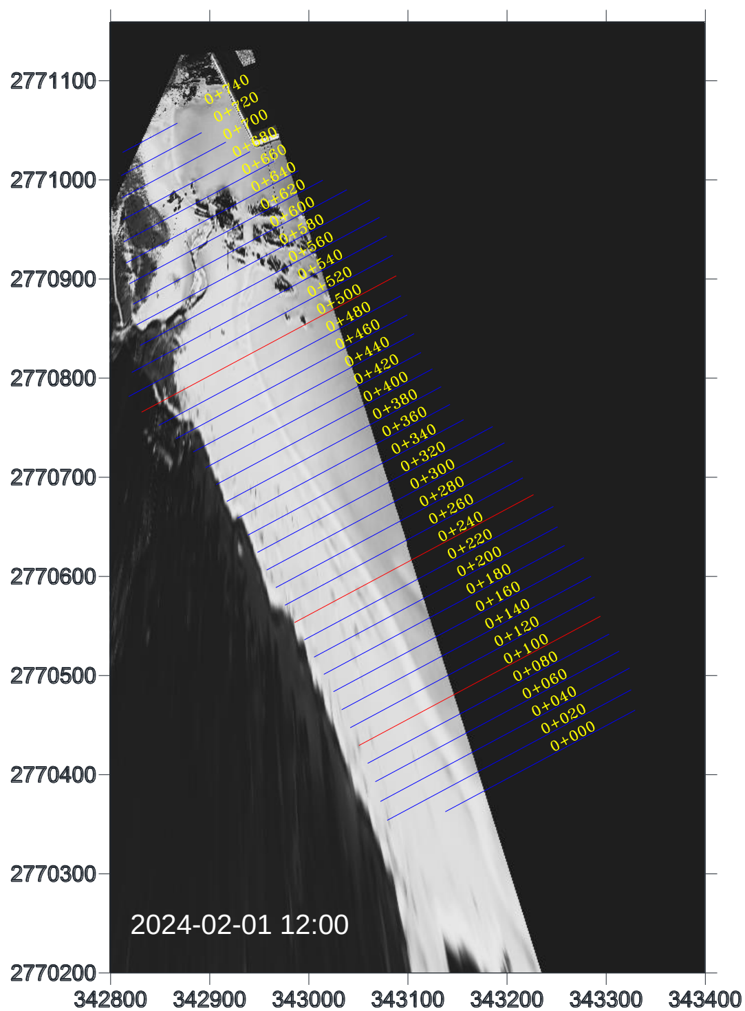
圖 4-19 鹽寮海岸地形影像全景圖(2024/02/01 12:00)
