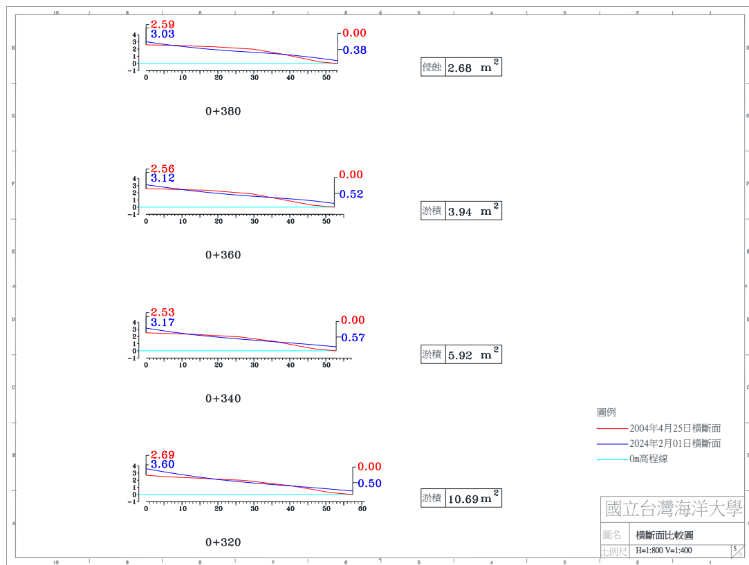
圖 4-4(f) 2024 年 2 月 1 日 A 監測區橫斷面比較圖
