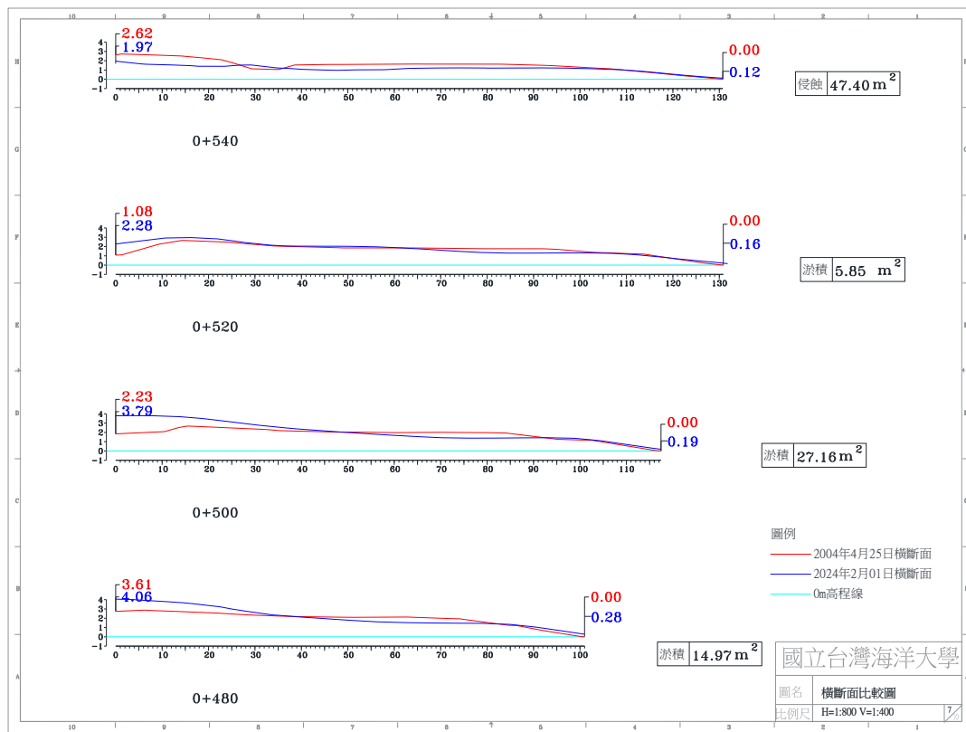
圖 4-4(d) 2024 年 2 月 1 日 A 監測區橫斷面比較圖
