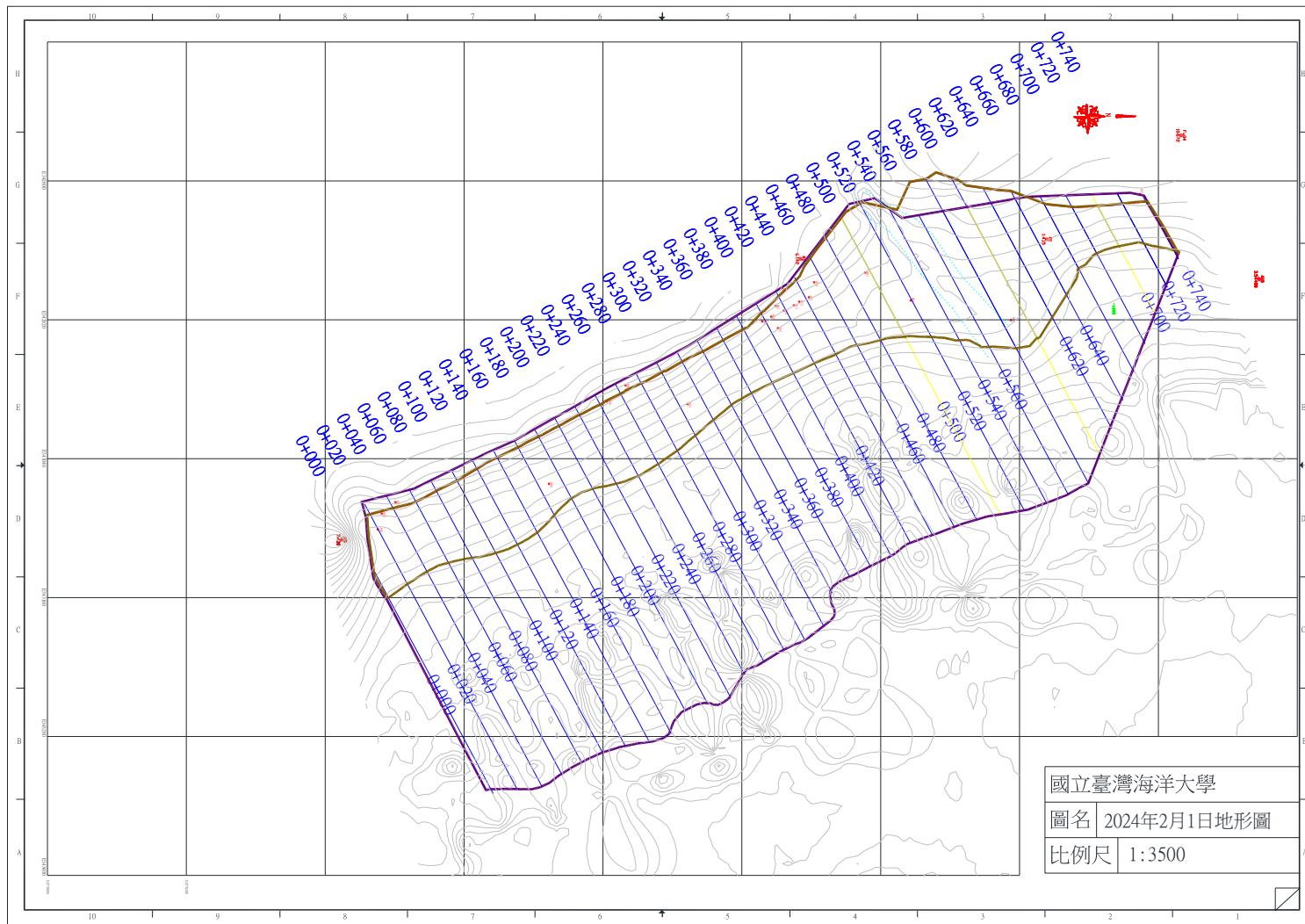
圖 4-1 2024 年 2 月 1 日監測地形
