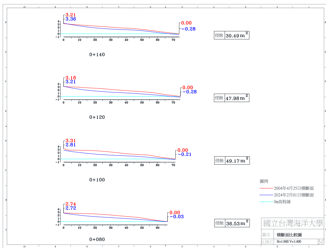
圖 4-4(i) 2024 年 2 月 1 日 A 監測區橫斷面比較圖
