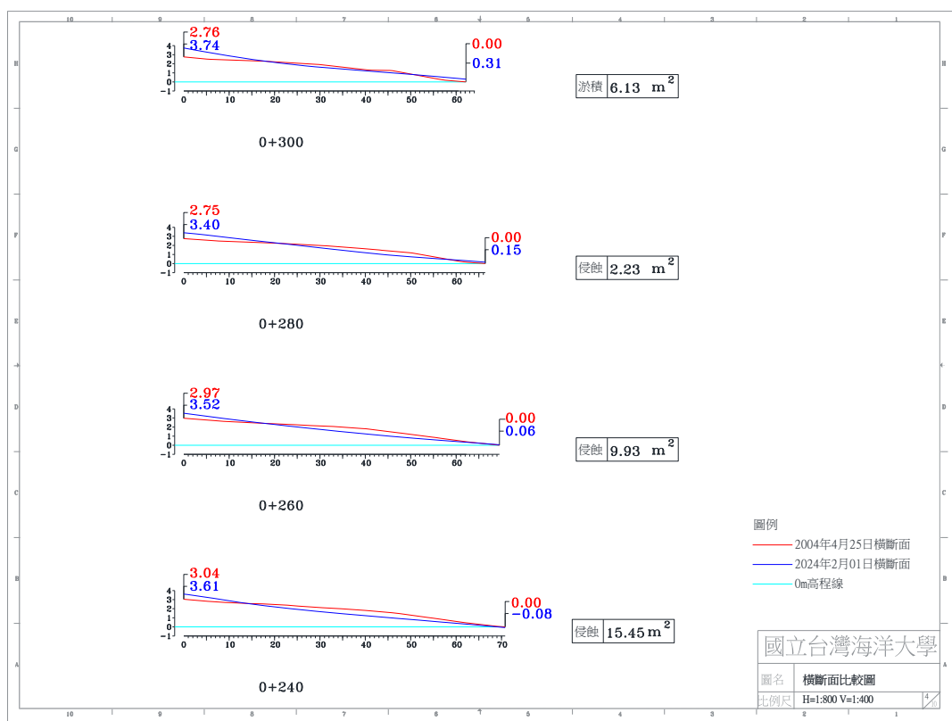
圖 4-4(g) 2024 年 2 月 1 日 A 監測區橫斷面比較圖
