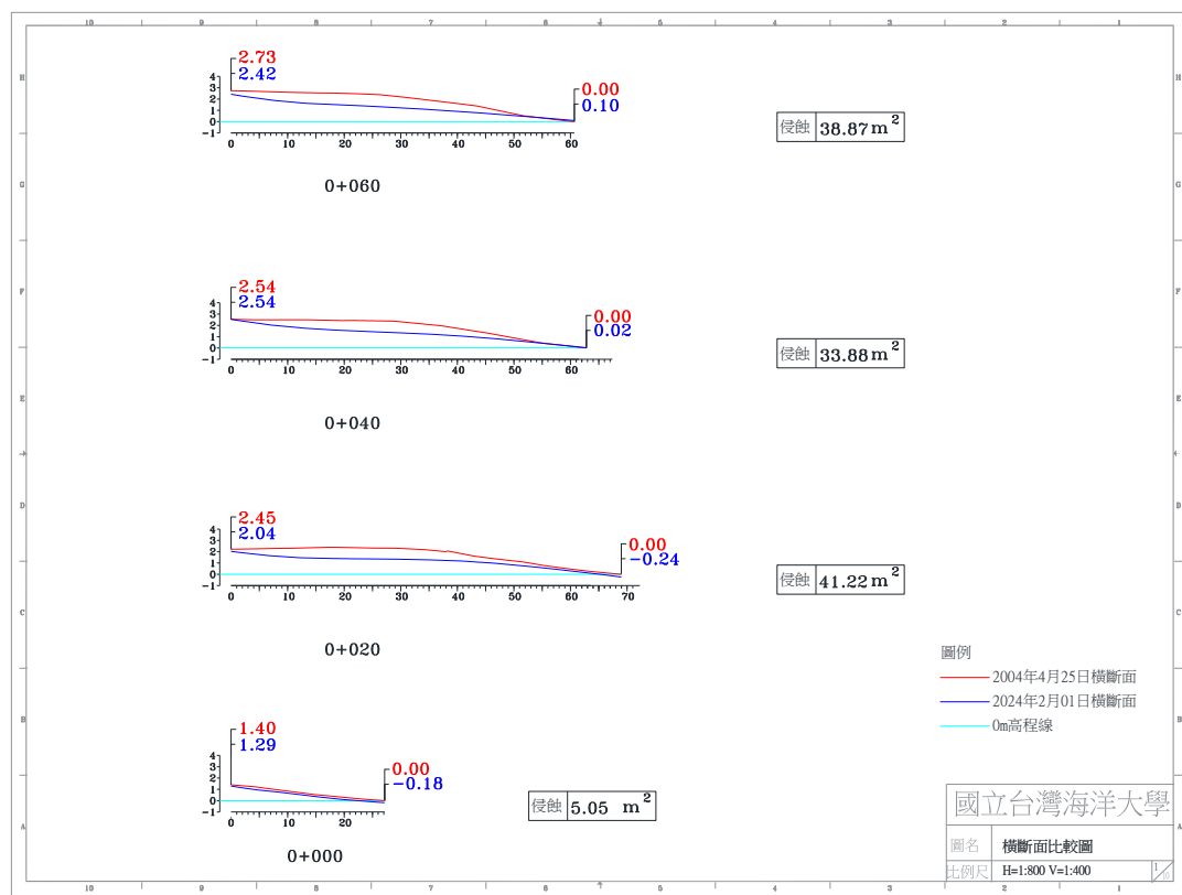
圖 4-4(j) 2024 年 2 月 1 日 A 監測區橫斷面比較圖
