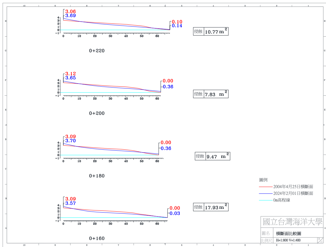
圖 4-4(h) 2024 年 2 月 1 日 A 監測區橫斷面比較圖
