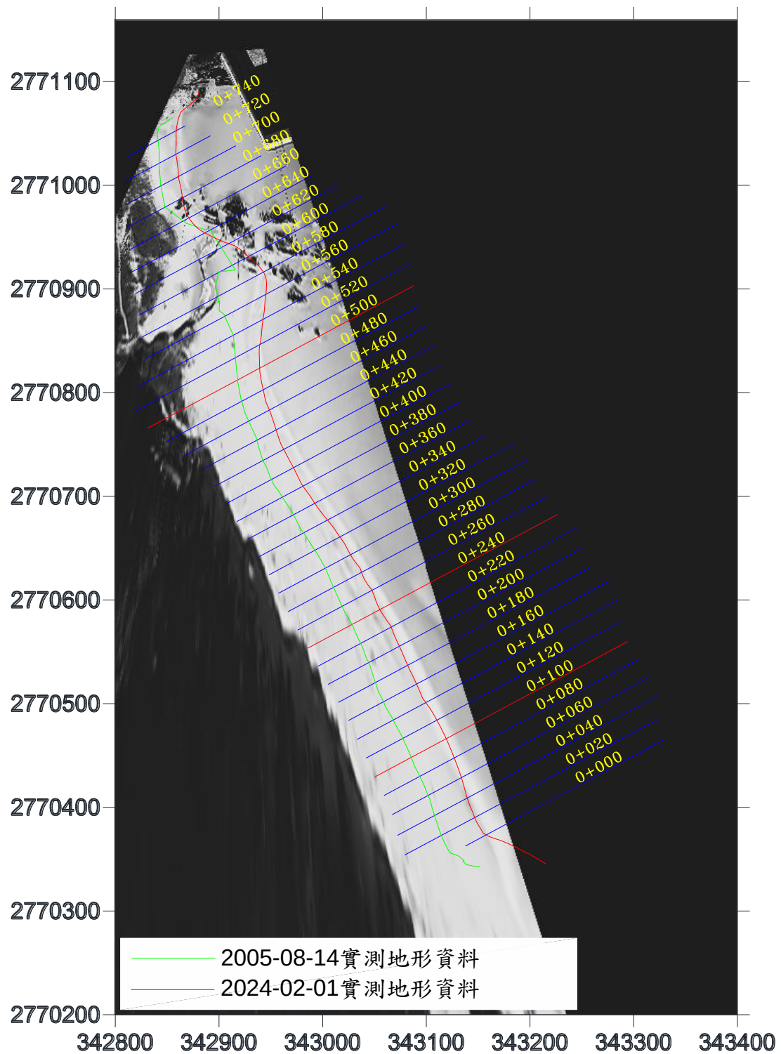
圖 4-22 長期實測 0 m 灘線比對平面示意圖
