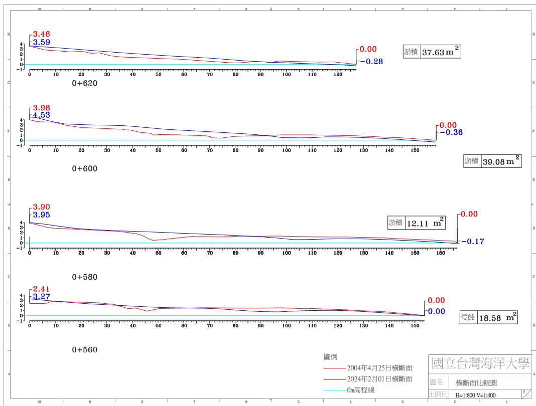
圖 4-4(c) 2024 年 2 月 1 日 A 監測區橫斷面比較圖
