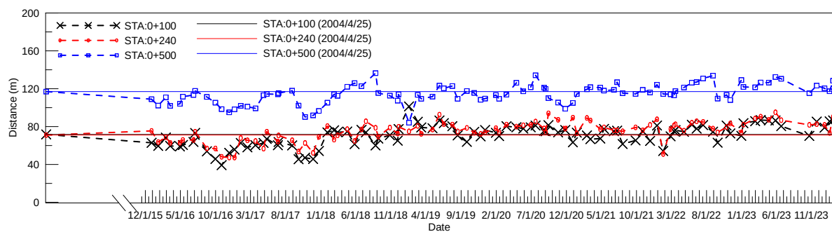
圖 4-21 岸線斷面沙灘寬度變化圖(2024/2/1)
