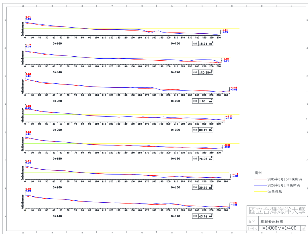
圖 4-5(e) 2024 年 2 月 1 日 B 監測區橫斷面比較圖
