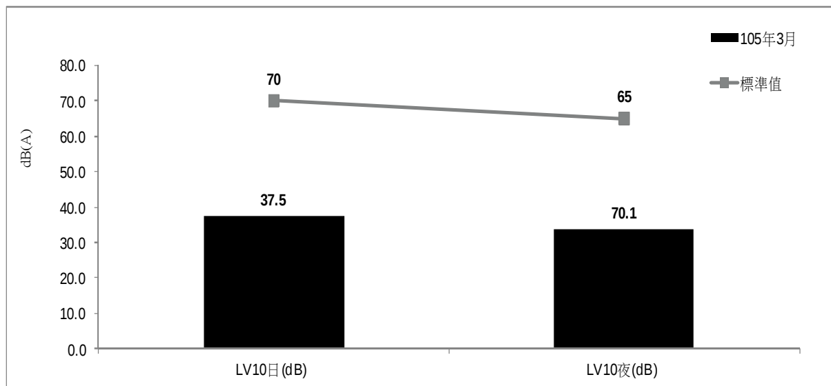
圖 2.2-2 計畫基地振動監測結果變化趨勢圖
