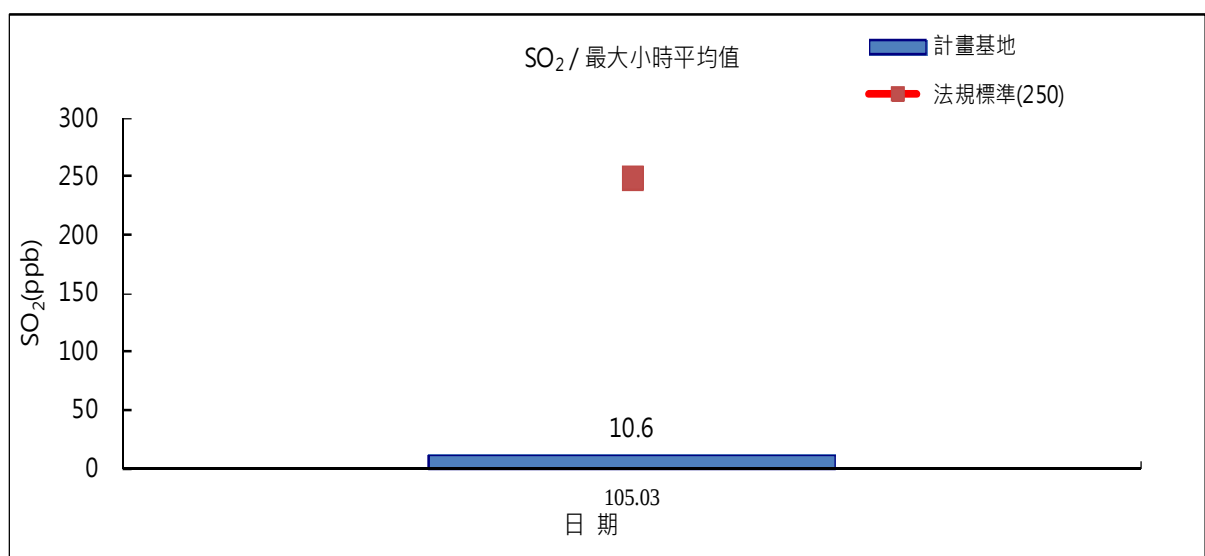
圖 2.1-1 空氣品質監測結果變化趨勢圖
