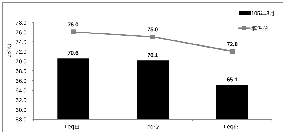
圖 2.2-1 計畫基地噪音監測結果變化趨勢圖
