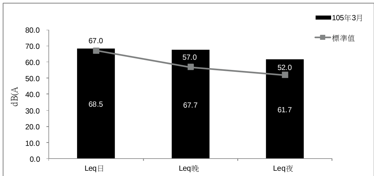
圖 2.3-1 出風口噪音監測結果變化趨勢圖
