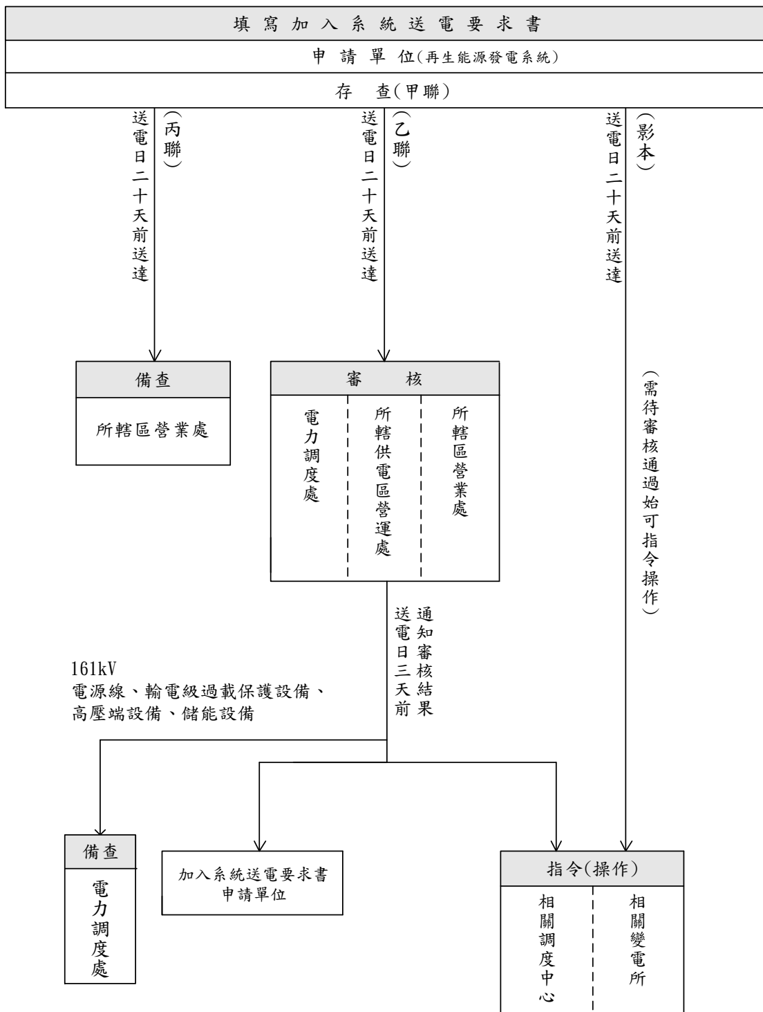
圖三：再生能源發電系統「加入系統送電要求書」作業流程圖
