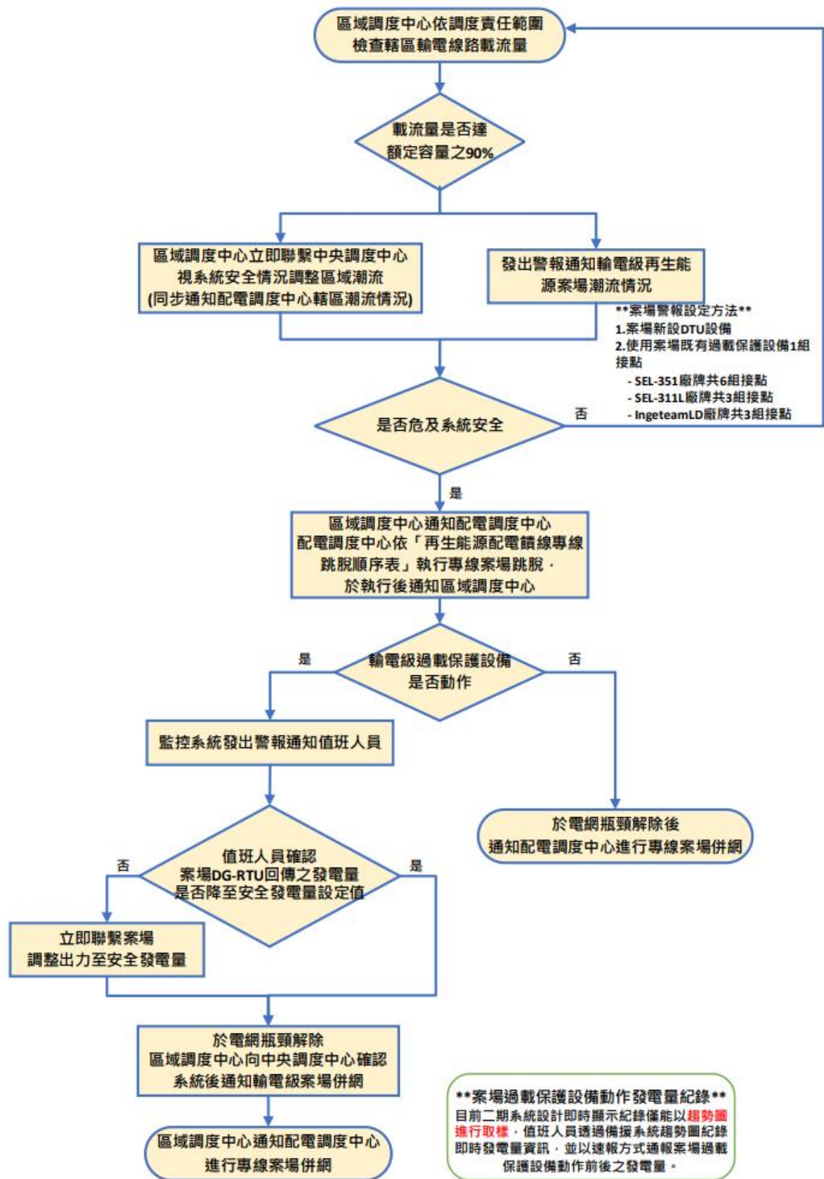
圖一：再生能源發電系統安全調度 流程示意圖(本島系統適用)
